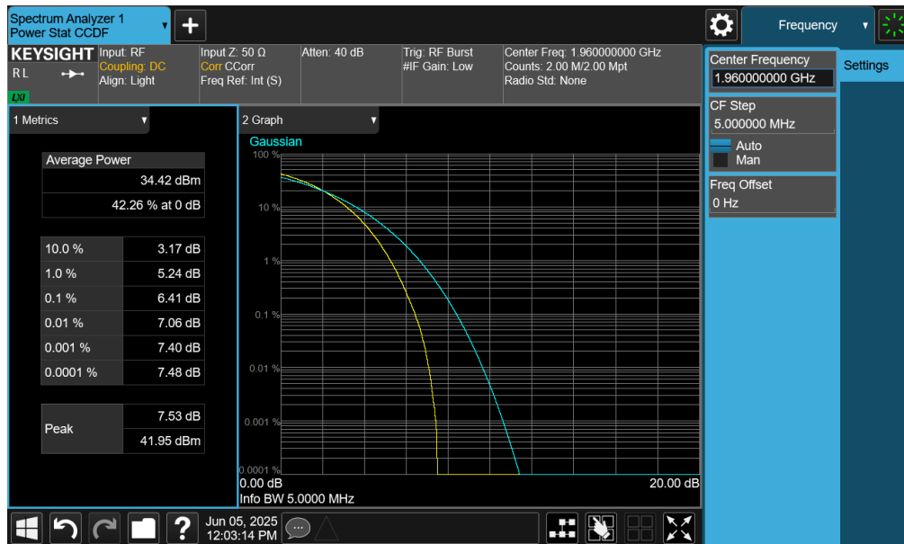
Plot 7-47. PAR Plot (WCDMA PCS)
