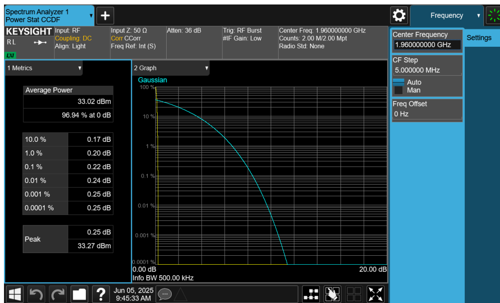
Plot 7-48. PAR Plot (GSM PCS)
