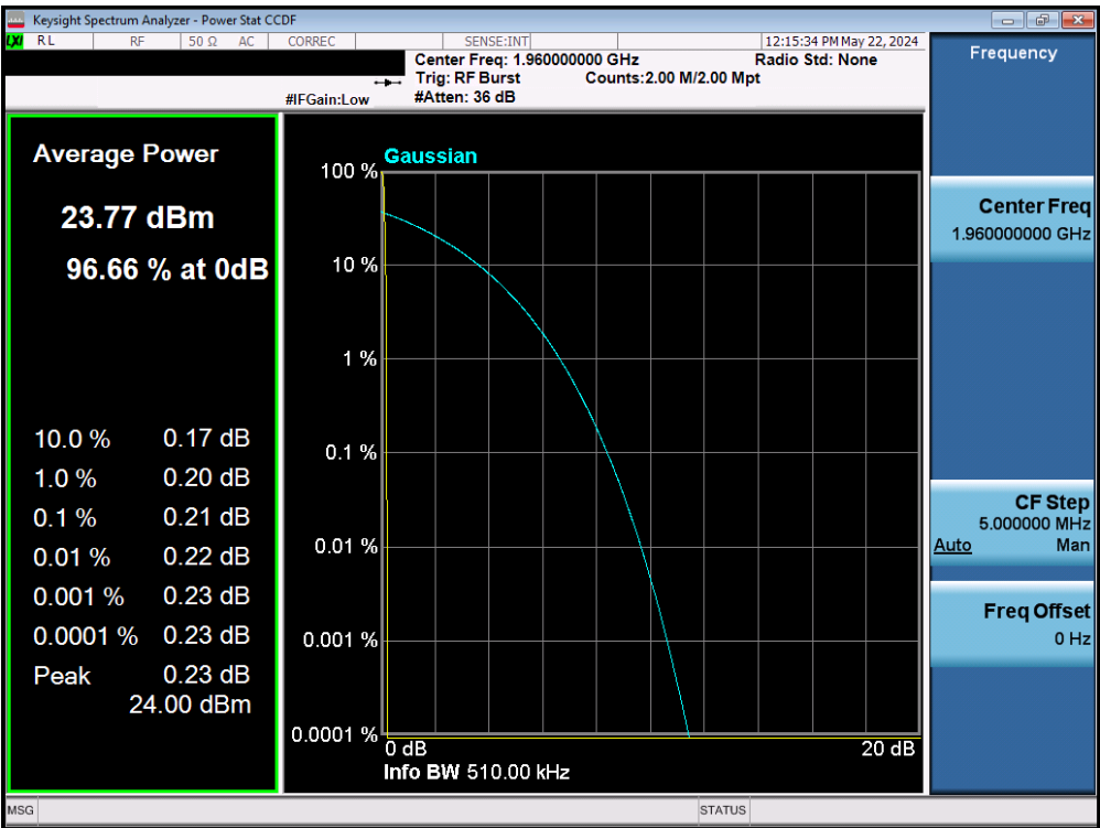
Plot 7-50. PAR Plot (GSM PCS)
