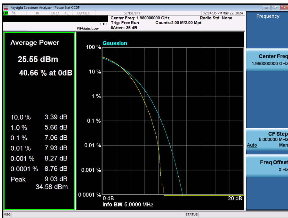
Plot 7-49. PAR Plot (WCDMA PCS)
