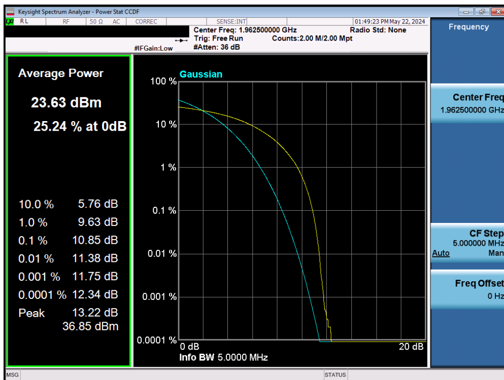
Plot 7-48. PAR Plot (LTE Band 25/2)
