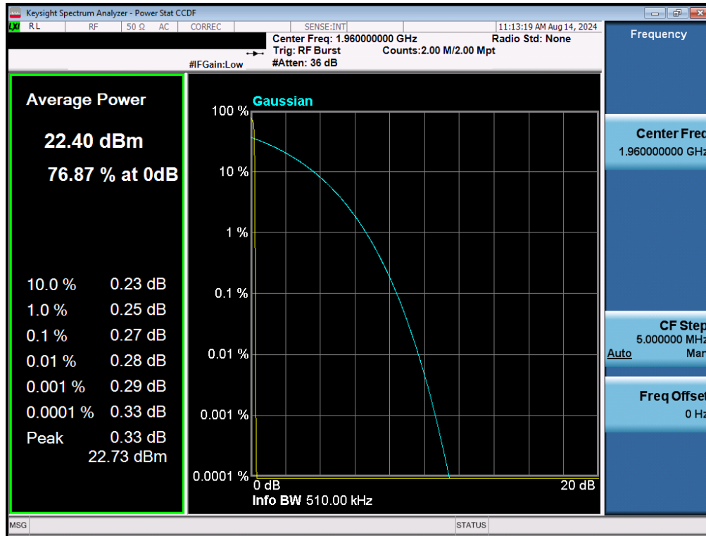
Plot 7-33. PAR Plot (GSM, Ch. 661)
