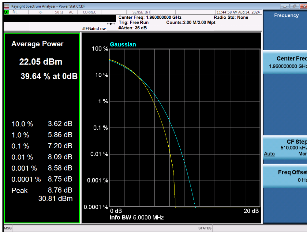
Plot 7-34. PAR Plot (UMTS, Ch. 9800)
