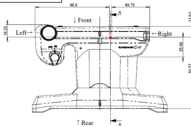
Top face
