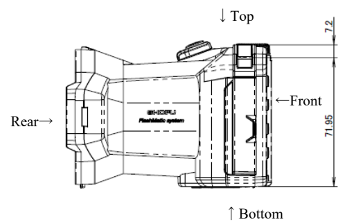
Right face
