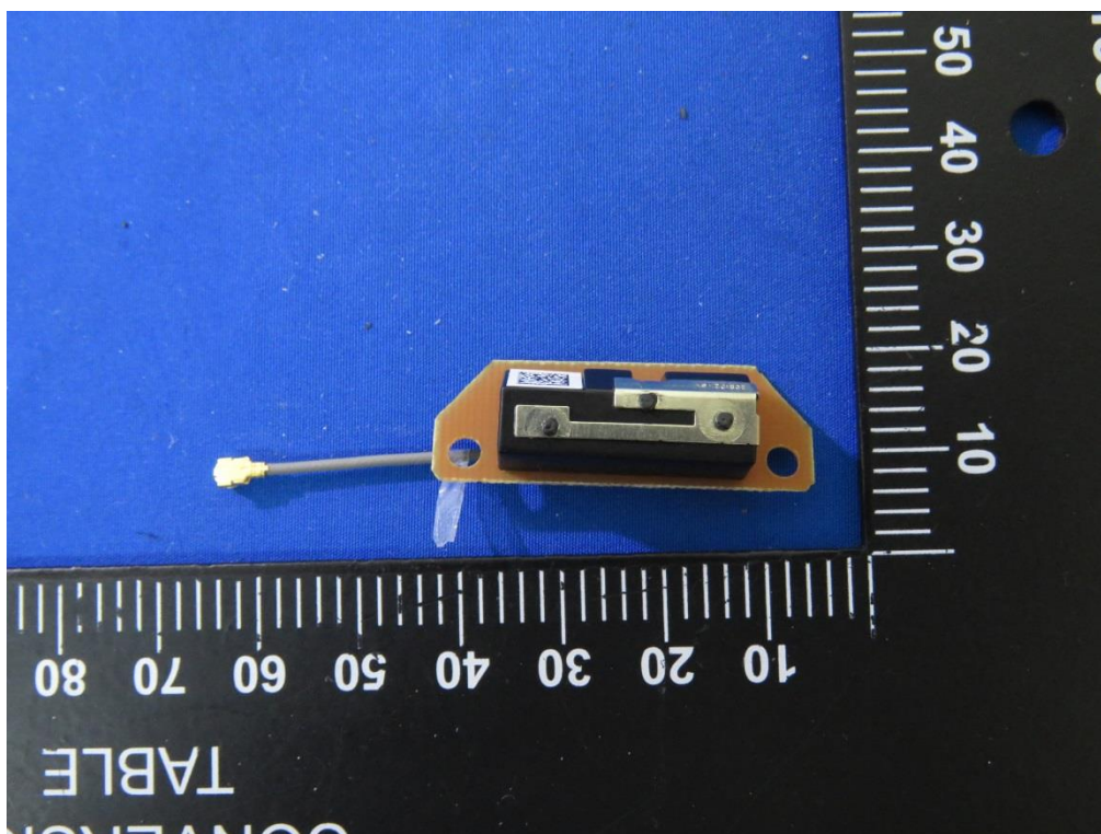
PIFA Antenna (SMARTEQ 4211613980)
