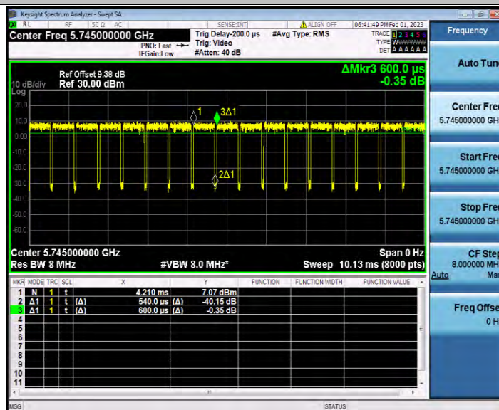
11AX20SISO_Ant3_5745
