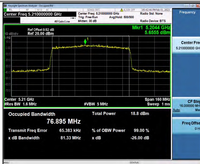
11AX80ISO_Ant3_5210
