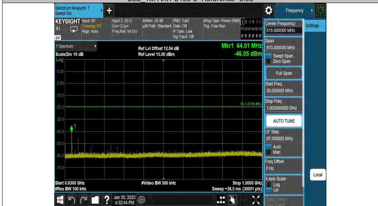
BLE 1M-Ant1-2480-30~1000--3.98
