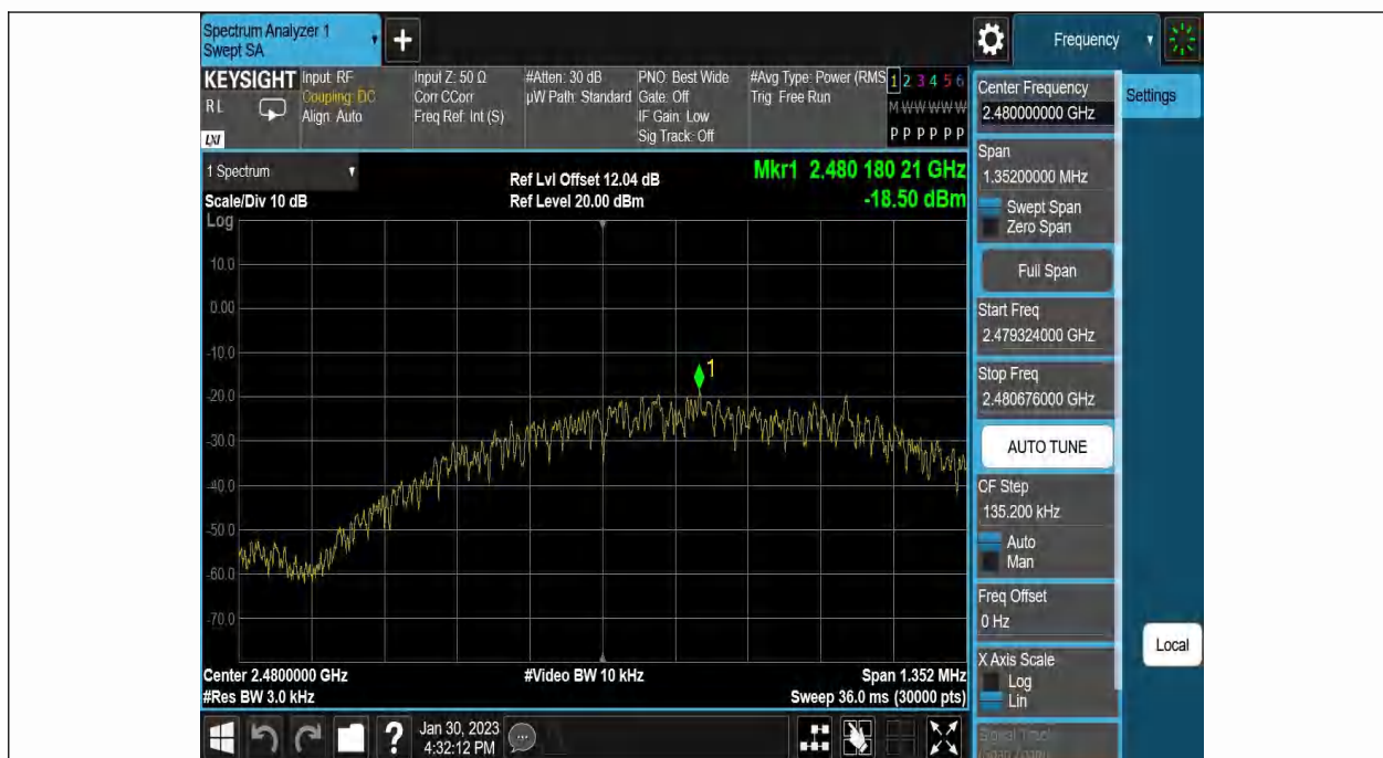
BLE 1M-Ant1-2480--18.50-0.00-0.00-0.00
