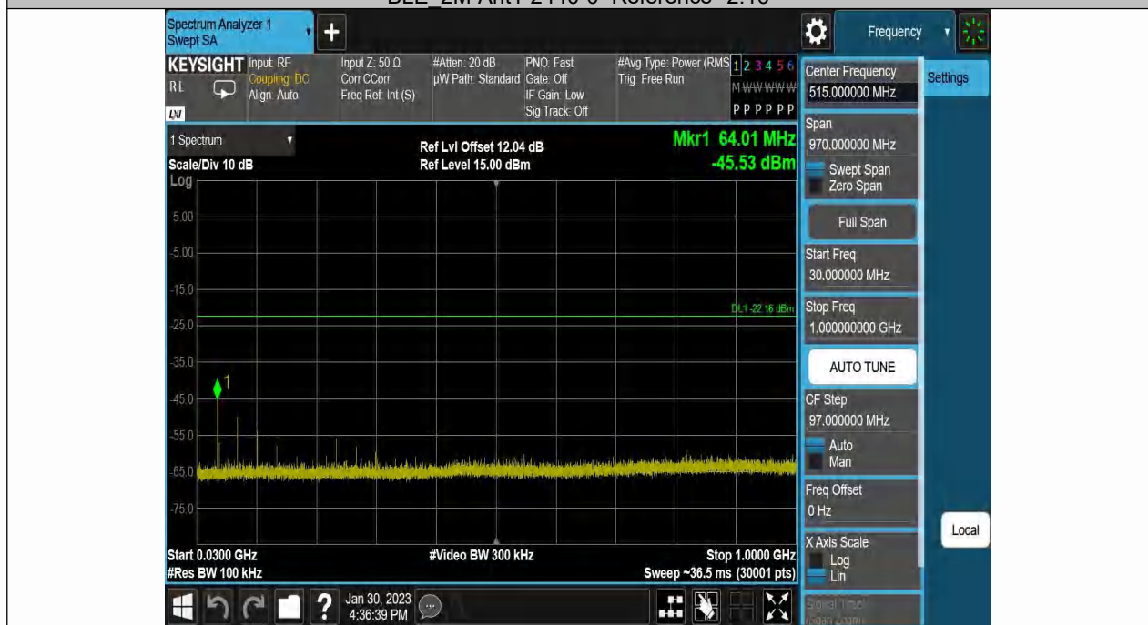
BLE 2M-Ant1-2440-30~1000--2.16
