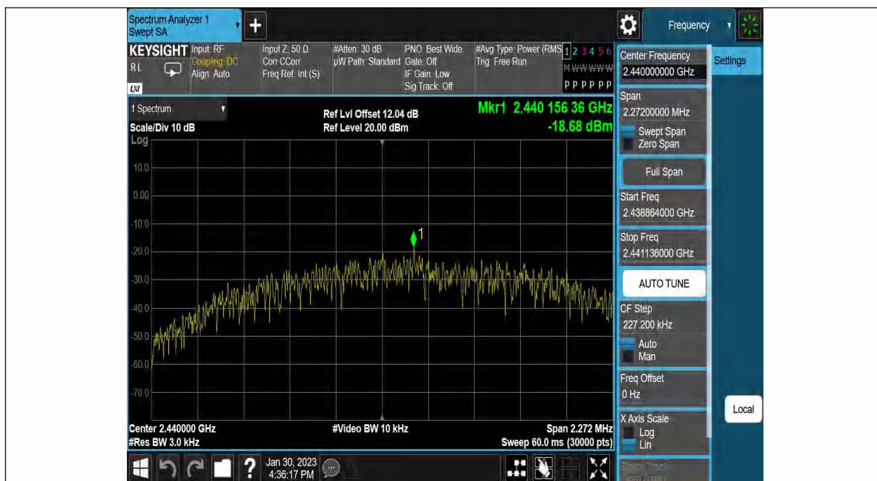
BLE 2M-Ant1-2440--18.68-0.00-0.00-0.00
