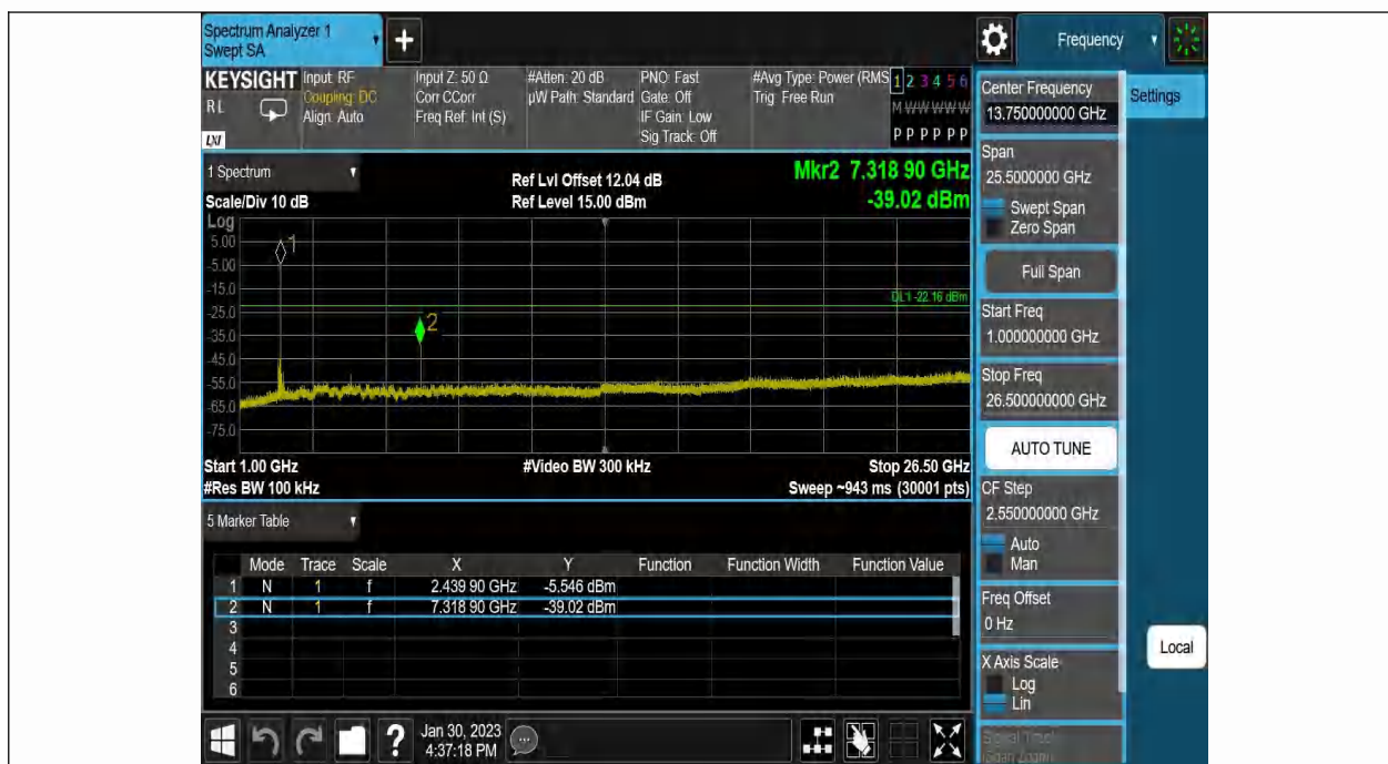
BLE_2M-Ant1-2440-1000~26500--2.16
