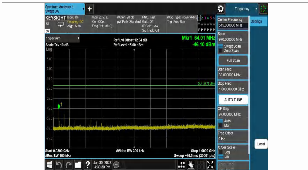
BLE_1M-Ant1-2440-30~1000--1.78
