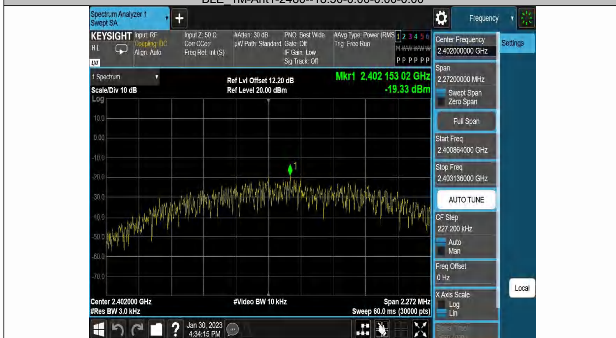
BLE 2M-Ant1-2402--19.33-0.00-0.00-0.00
