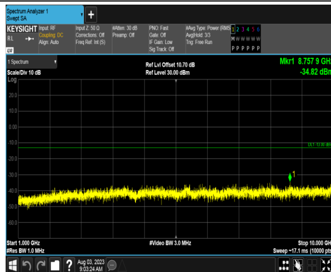
Band26B-1.4MHz-QPSK-26697-1RB#0-Range2:1000~10000MHz
