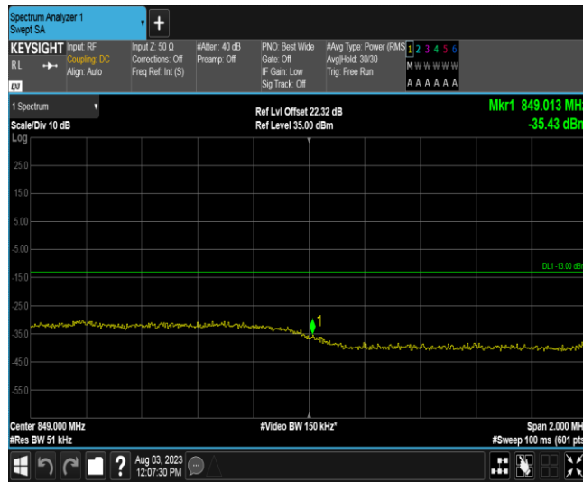
Band26A-3MHz-QPSK-27025-1RB#14
