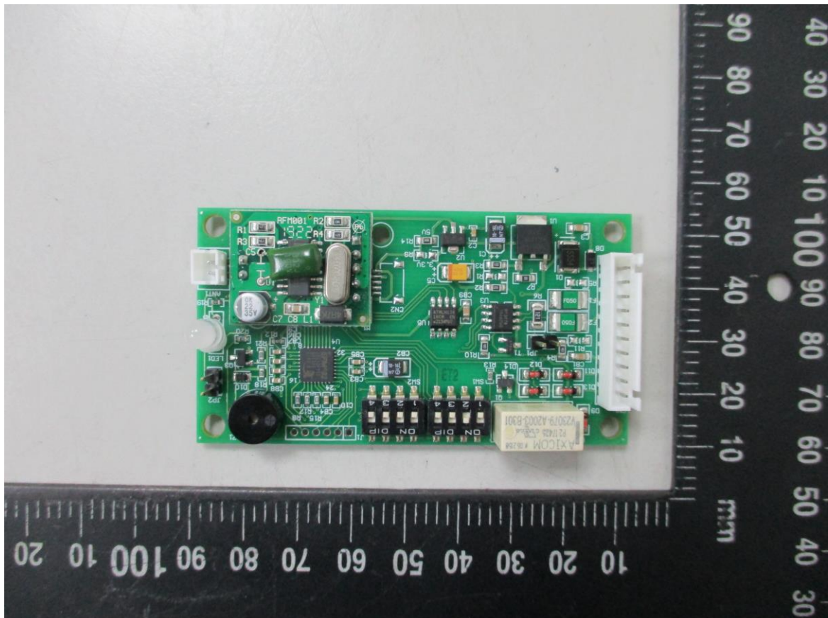
RFID Module 2
