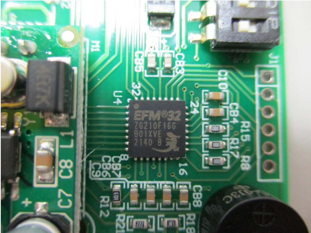
RFID Module 2
