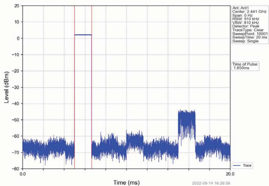
GFSK_DH3_HOPP_Ant1_NTNV
