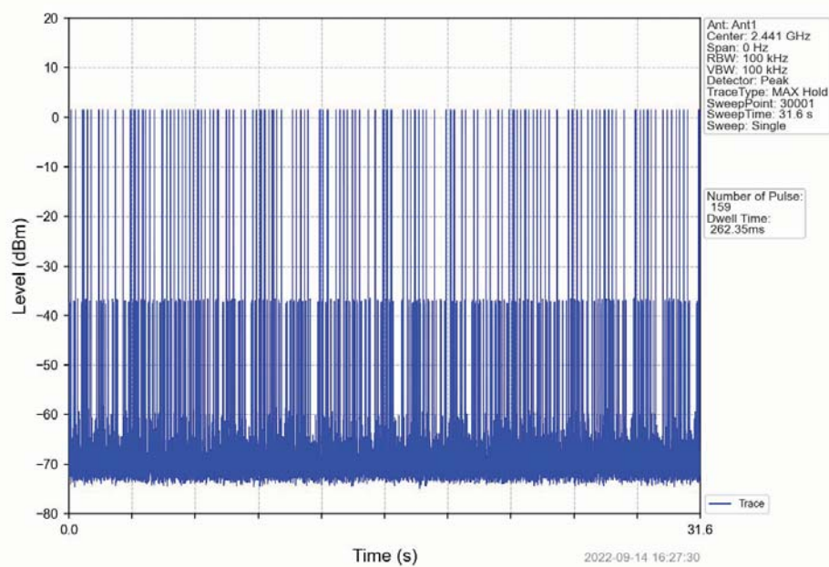
GFSK_DH3_HOPP_Ant1_NTNV
