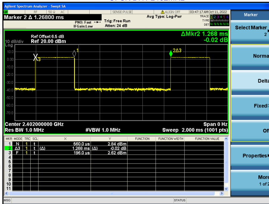
GFSK DH1 2402MHz
