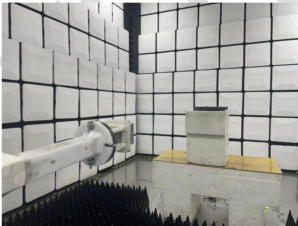
Above 18GHz Horizontal
