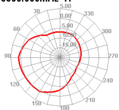
5500.000MHz H
