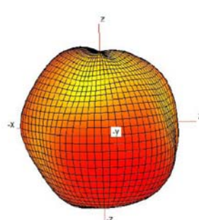
2200MHz
