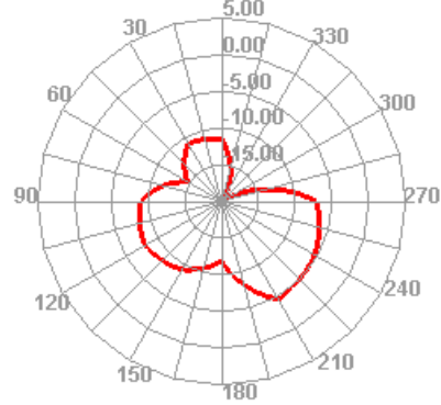
888.000MHz E2
