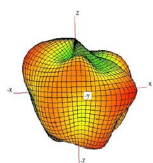
960MHz
