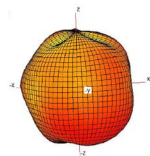
2600MHz
