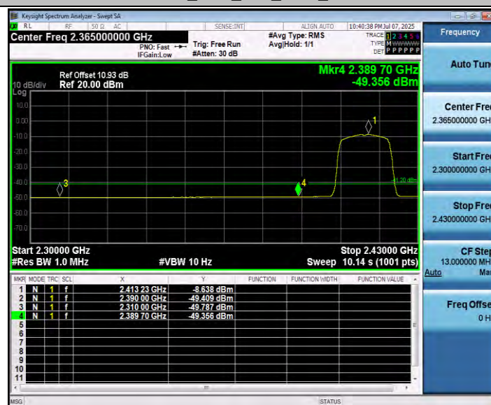
11G_Ant2_Low_2412_AV
