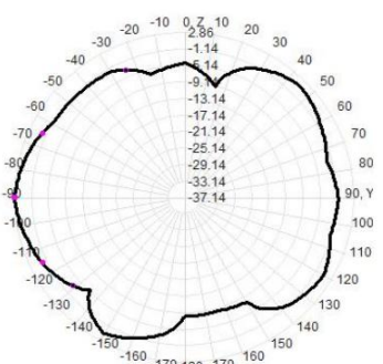
5850MHz
