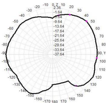
5550MHz
