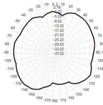
5150MHz
