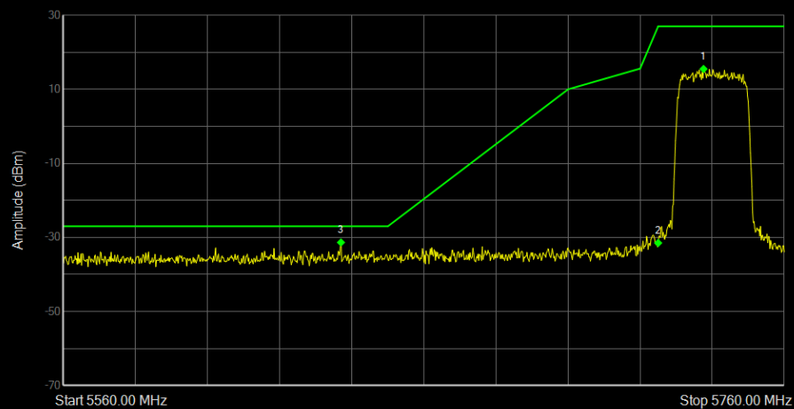
Band Edge NVNT 20M 5740MHz Low Ant 2
