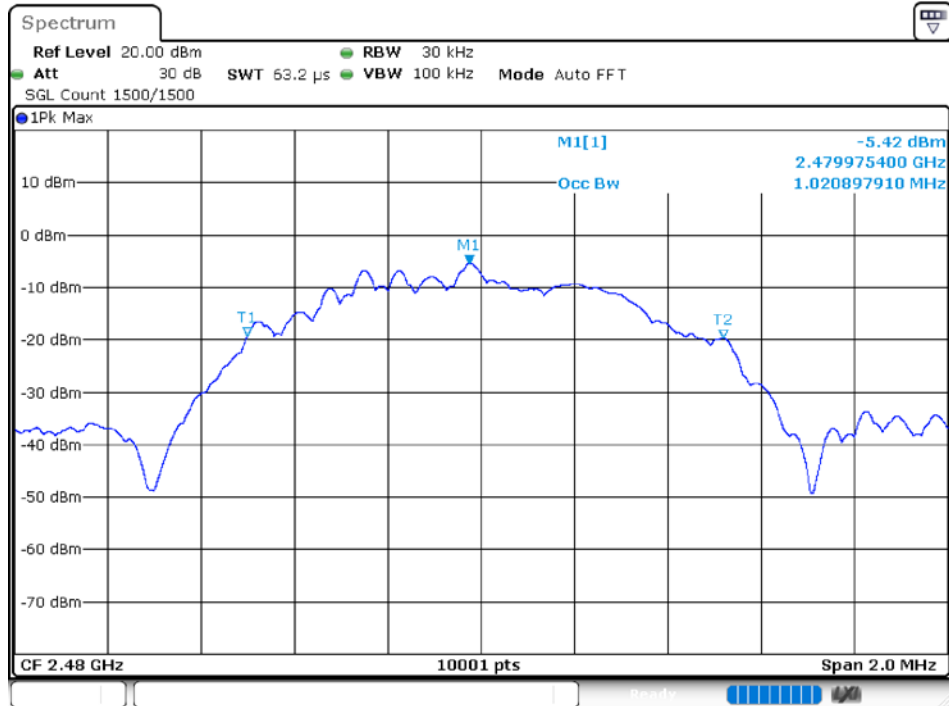
-6 dB BW NVNT BLE 2480MHz Ant1
