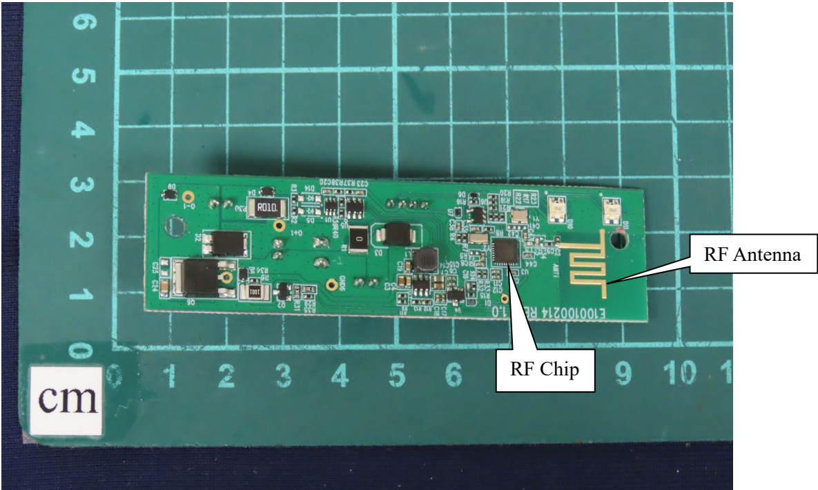
(15) EUT Photo
