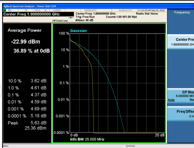
Band2-20MHz-16QAM-19100-100RB#0
