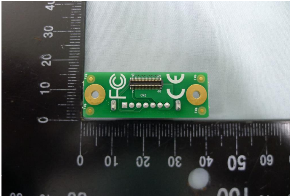
(20) EUT Photo
