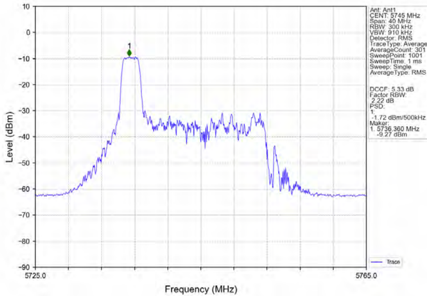
802.11ax(HEW20)_LCH_5745MHz_RU26_Left_Ant1_NTNV
