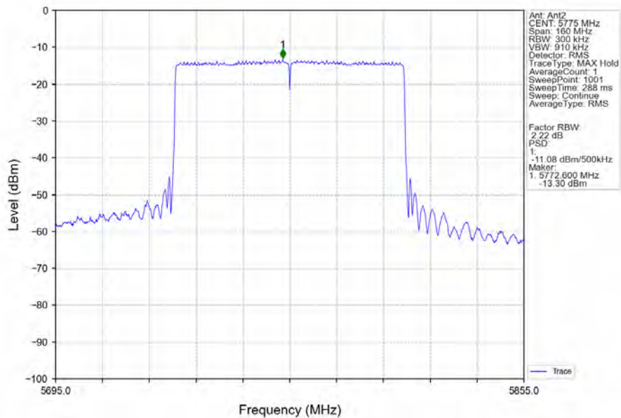
802.11ax(HEW80)_MCH_5775MHz_RU996_Left_Ant2_NTNV
