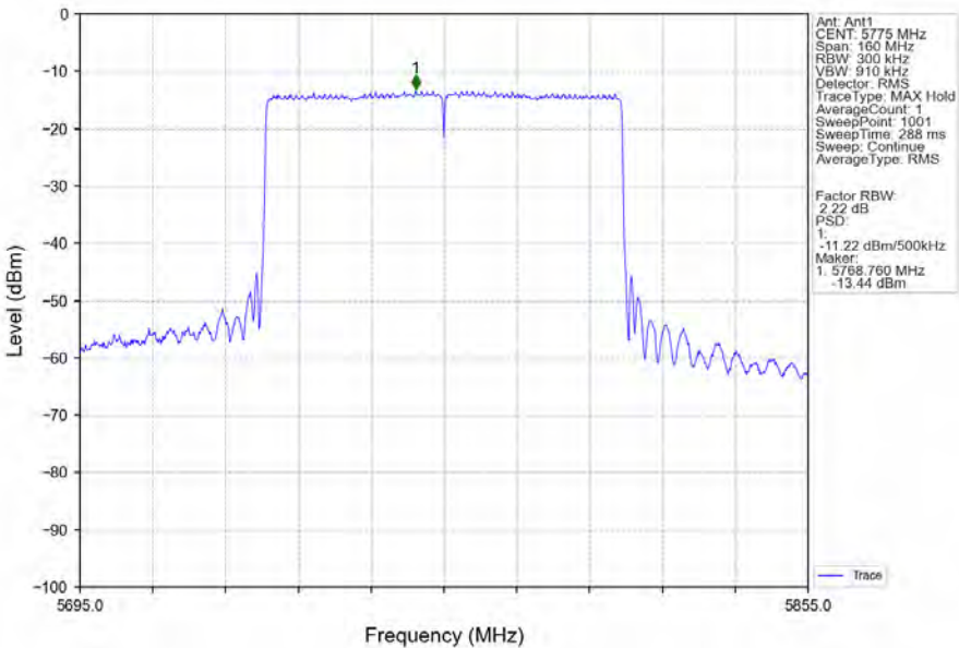
802.11ax(HEW80)_MCH_5775MHz_RU996_Left_Ant1_NTNV
