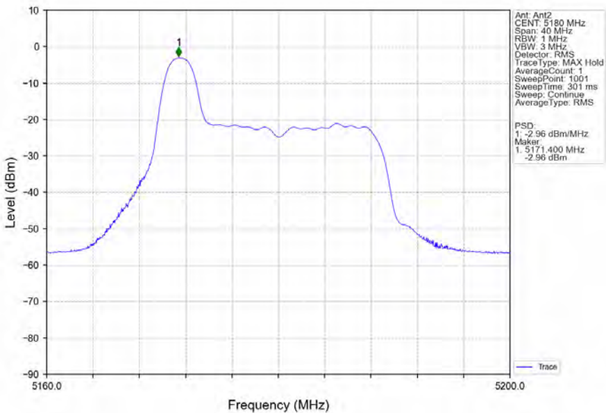
802.11ax(HEW20)_LCH_5180MHz_RU26_Left_Ant2_NTNV
