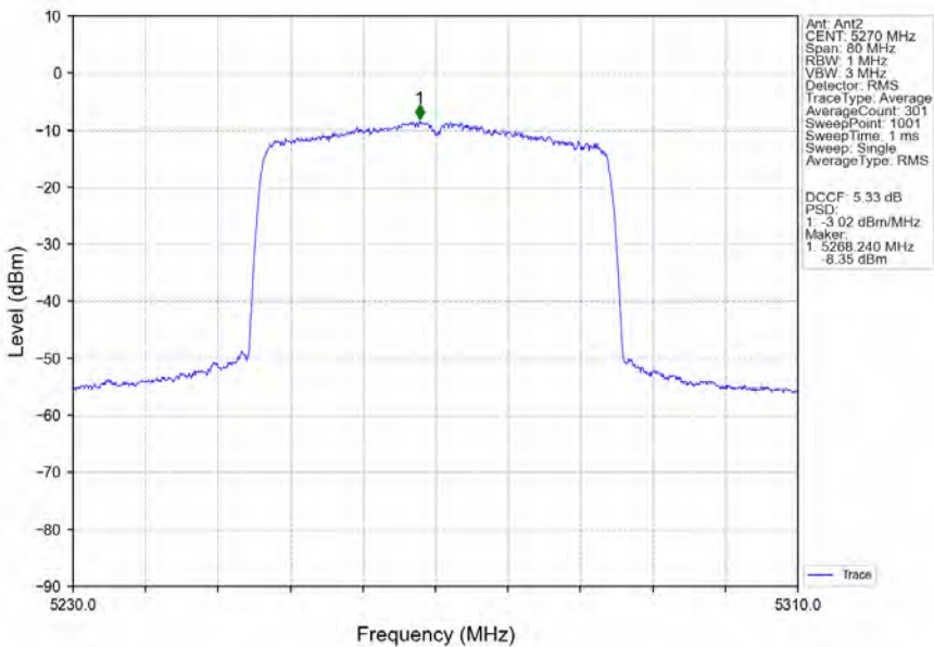
802.11ax(HEW40)_LCH_5270MHz_RU484_Left_Ant2_NTNV
