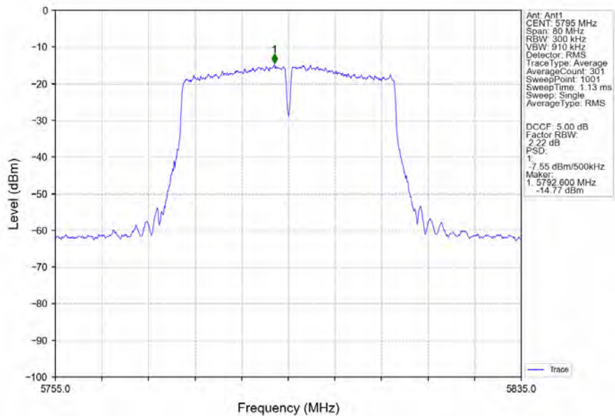
802.11n(HT40)_HCH_5795MHz_Ant1_NTNV
