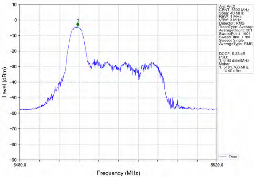
802.11ax(HEW20)_LCH_5500MHz_RU26_Left_Ant2_NTNV
