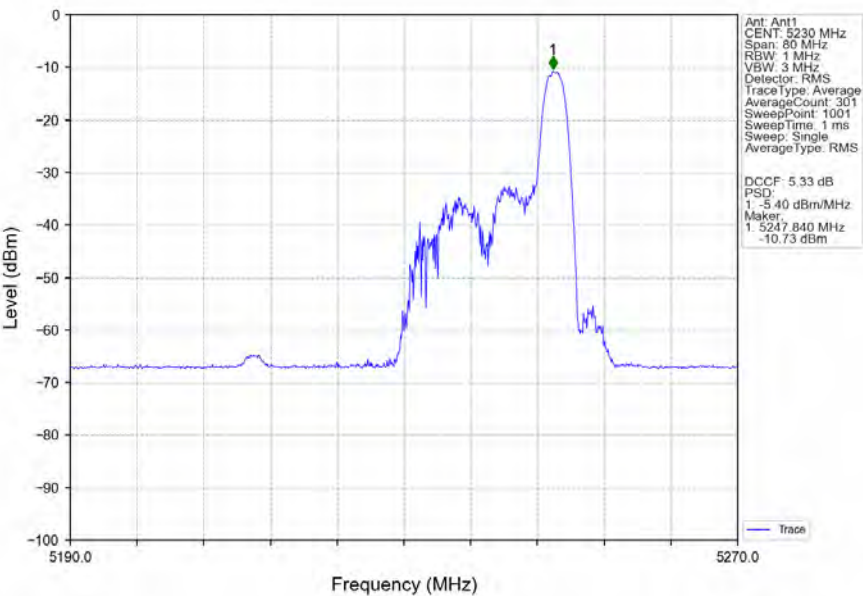
802.11ax(HEW40)_HCH_5230MHz_RU26_Right_Ant1_NTNV
