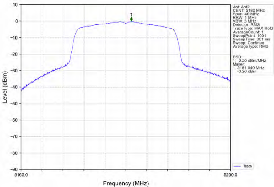
802.11ax(HEW20)_LCH_5180MHz_RU242_Left_Ant2_NTNV
