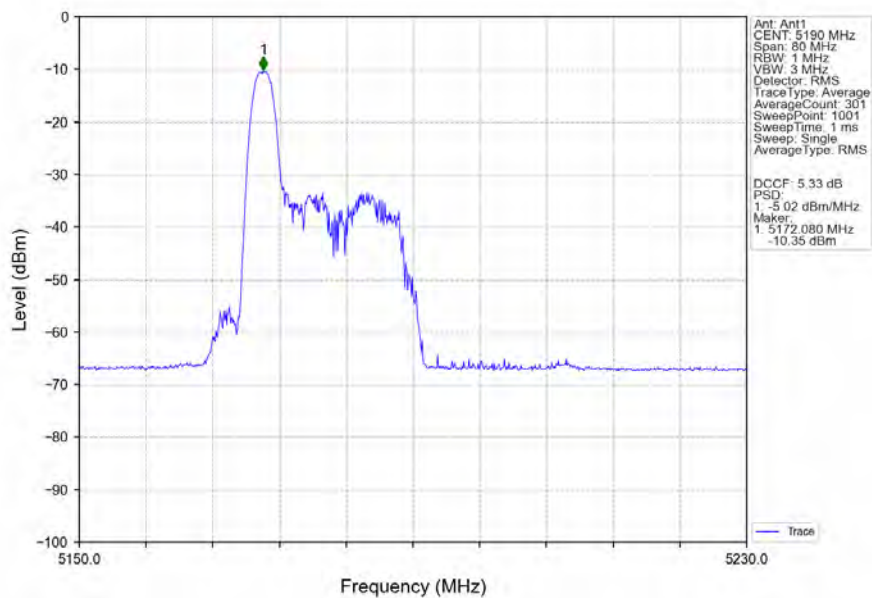
802.11ax(HEW40)_LCH_5190MHz_RU26_Left_Ant1_NTNV
