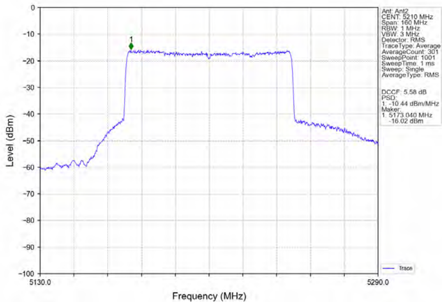
802.11ax(HEW80)_MCH_5210MHz_RU996_Left_Ant2_NTNV
