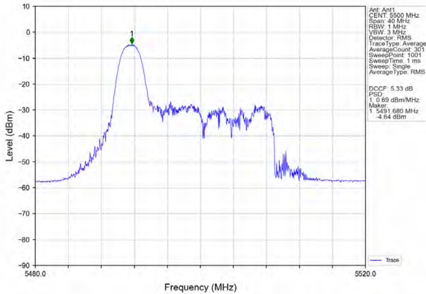
802.11ax(HEW20)_LCH_5500MHz_RU26_Left_Ant1_NTNV
