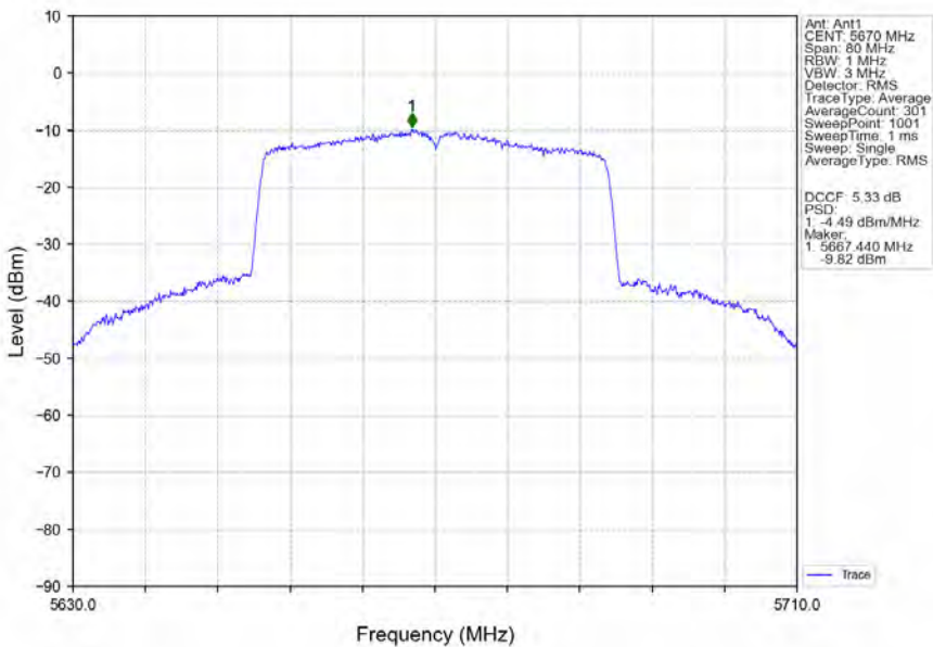
802.11ax(HEW40)_HCH_5670MHz_RU484_Left_Ant1_NTNV
