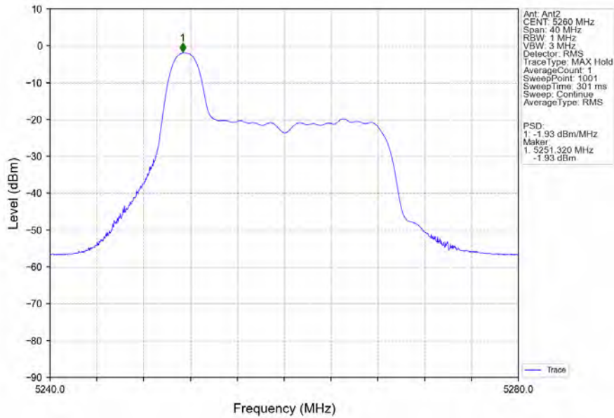
802.11ax(HEW20)_LCH_5260MHz_RU26_Left_Ant2_NTNV
