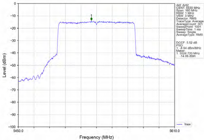
802.11ax(HEW80)_LCH_5530MHz_RU996_Left_Ant2_NTNV
