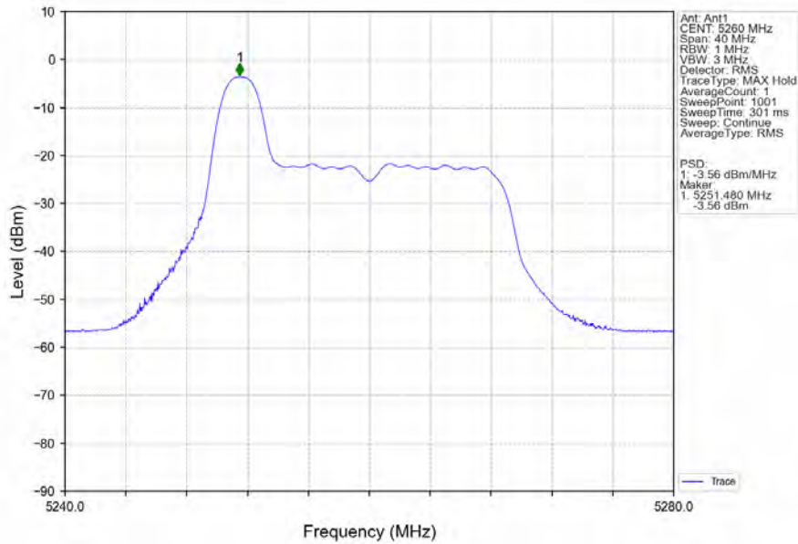
802.11ax(HEW20)_LCH_5260MHz_RU26_Left_Ant1_NTNV
