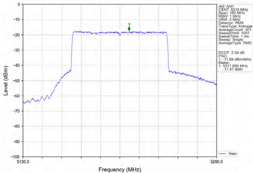
802.11ax(HEW80)_MCH_5210MHz_RU996_Left_Ant1_NTNV
