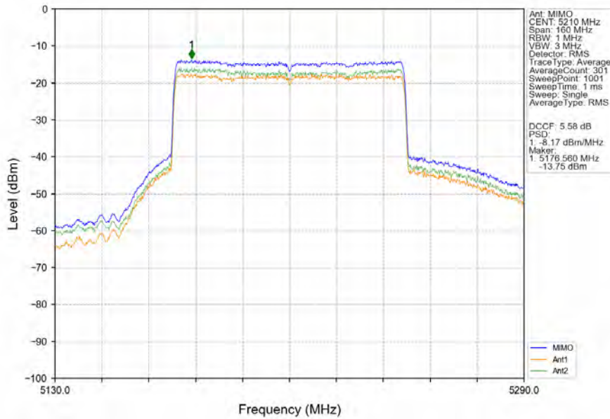
802.11ax(HEW80)_MCH_5210MHz_RU996_Left_MIMO_NTNV
