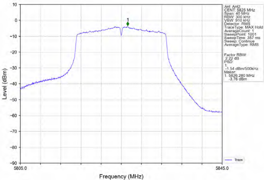
802.11n(HT20)_HCH_5825MHz_Ant2_NTNV
