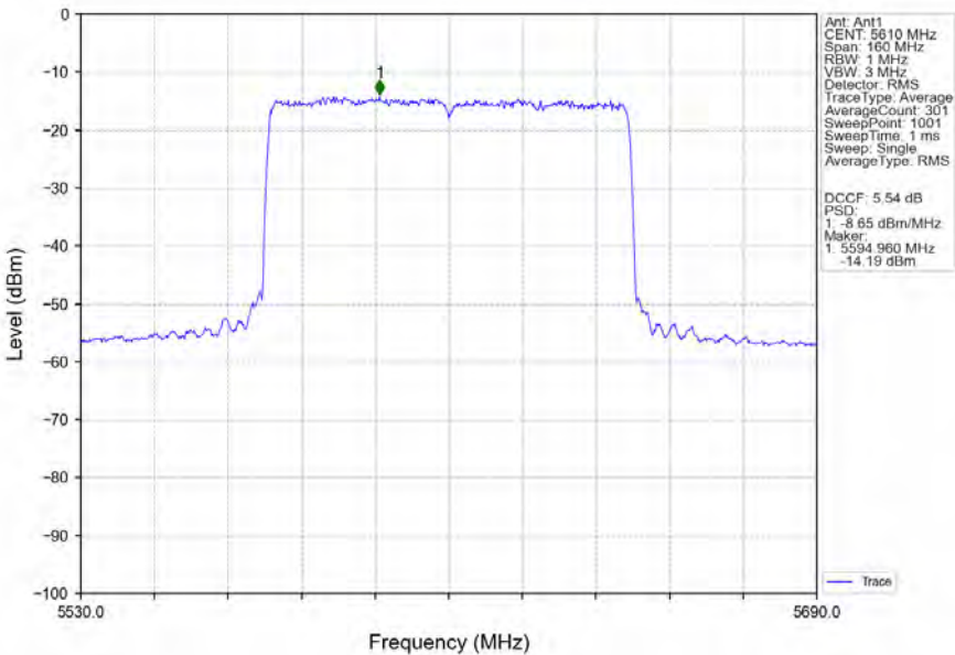
802.11ax(HEW80)_HCH_5610MHz_RU996_Left_Ant1_NTNV
