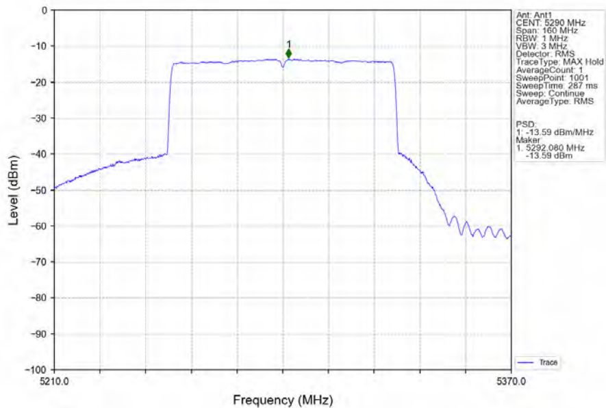
802.11ax(HEW80)_MCH_5290MHz_RU996_Left_Ant1_NTNV
