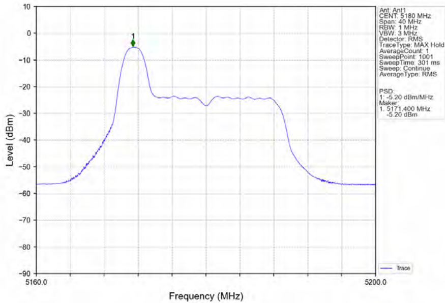
802.11ax(HEW20)_LCH_5180MHz_RU26_Left_Ant1_NTNV
