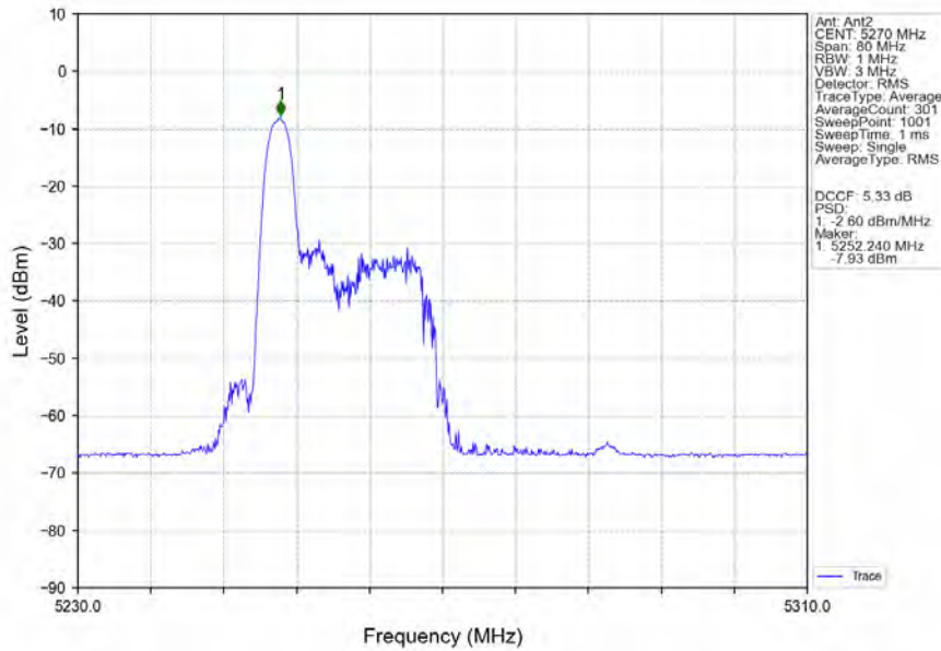
802.11ax(HEW40)_LCH_5270MHz_RU26_Left_Ant2_NTNV
