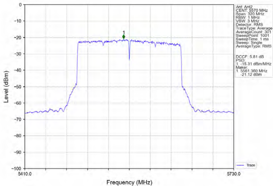
802.11ax(HEW160)_MCH_5570MHz_2xRU996_Left_Ant2_NTNV
