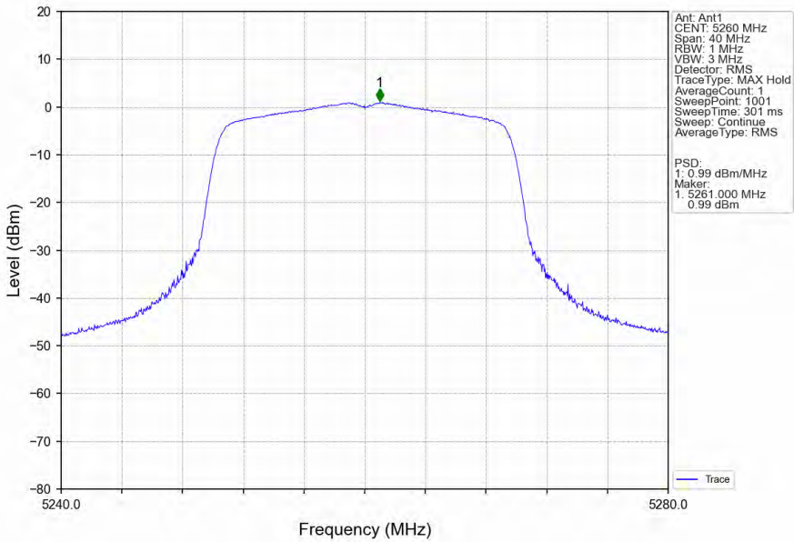
802.11ax(HEW20)_LCH_5260MHz_RU242_Left_Ant1_NTNV
