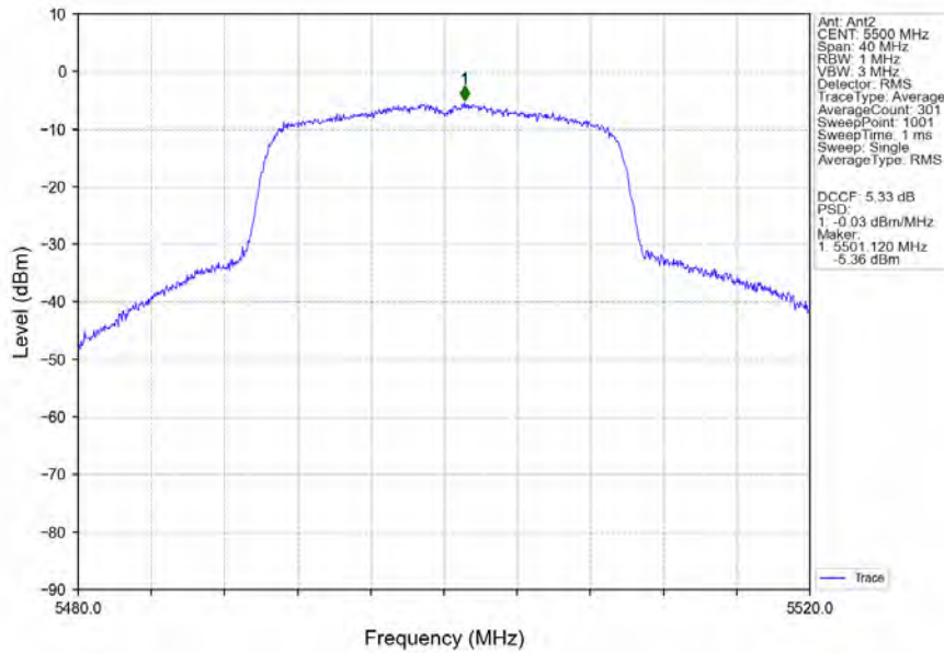
802.11ax(HEW20)_LCH_5500MHz_RU242_Left_Ant2_NTNV
