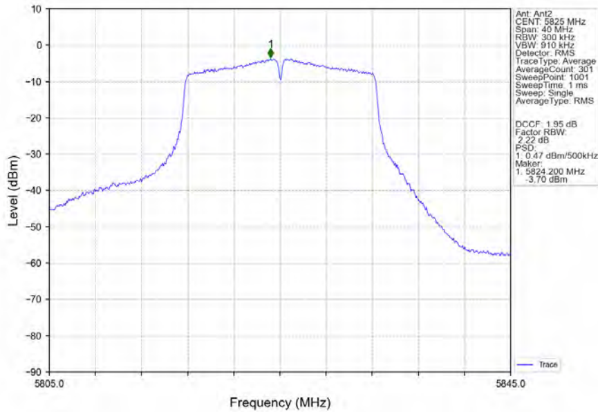
802.11a_HCH_5825MHz_Ant2_NTNV
