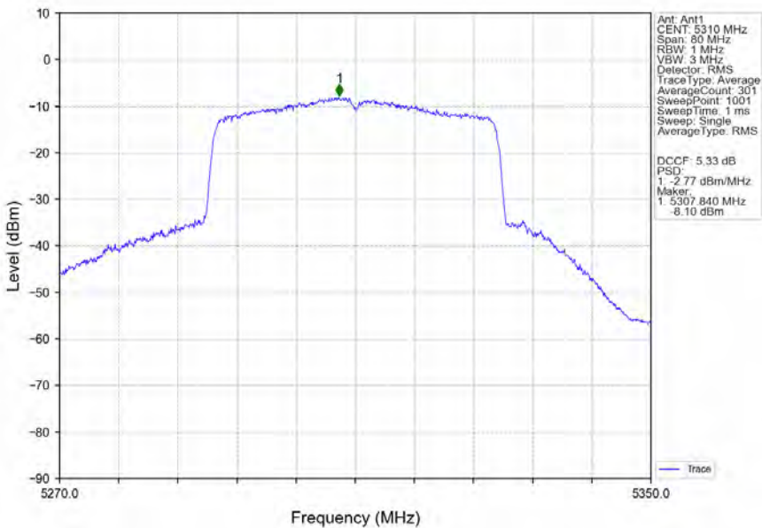
802.11ax(HEW40)_HCH_5310MHz_RU484_Left_Ant1_NTNV
