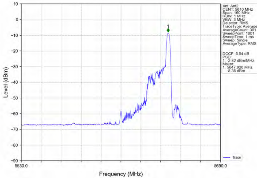
802.11ax(HEW80)_HCH_5610MHz_RU26_Right_Ant2_NTNV
