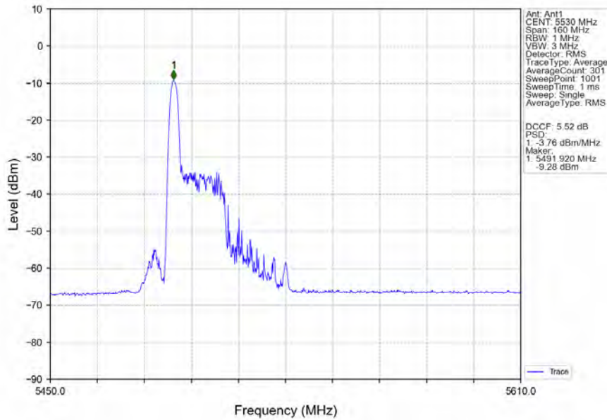
802.11ax(HEW80)_LCH_5530MHz_RU26_Left_Ant1_NTNV
