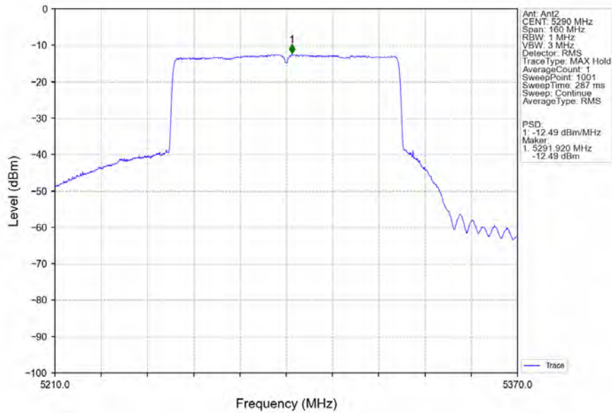
802.11ax(HEW80)_MCH_5290MHz_RU996_Left_Ant2_NTNV
