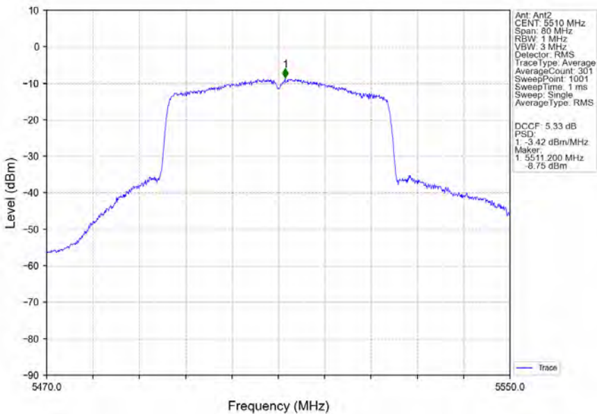
802.11ax(HEW40)_LCH_5510MHz_RU484_Left_Ant2_NTNV
