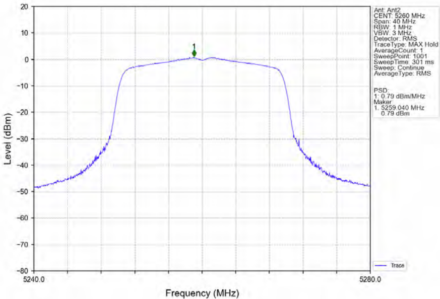
802.11ax(HEW20)_LCH_5260MHz_RU242_Left_Ant2_NTNV
