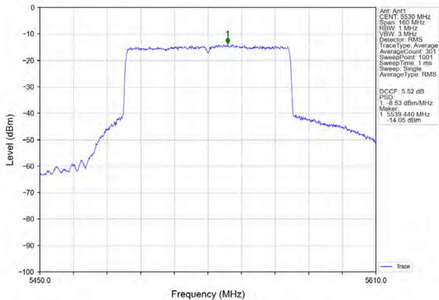
802.11ax(HEW80)_LCH_5530MHz_RU996_Left_Ant1_NTNV
