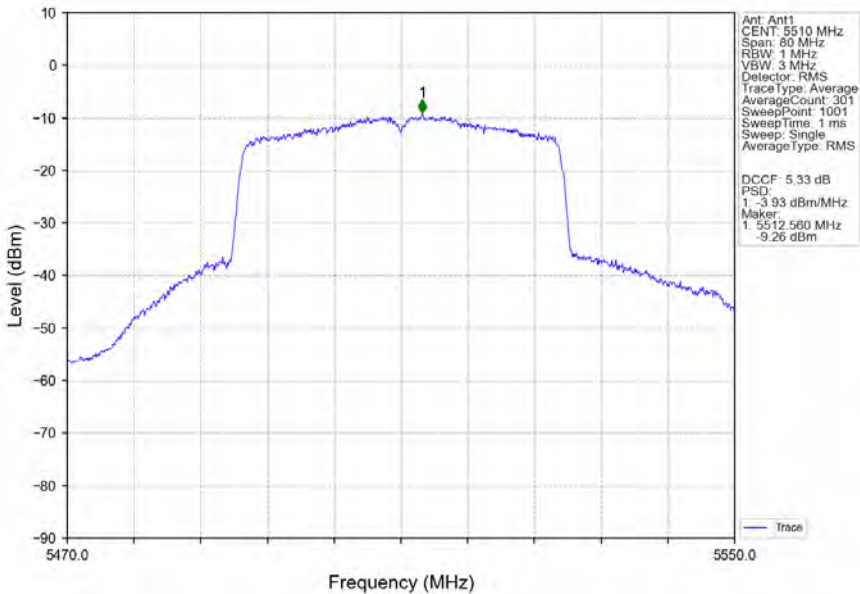
802.11ax(HEW40)_LCH_5510MHz_RU484_Left_Ant1_NTNV
