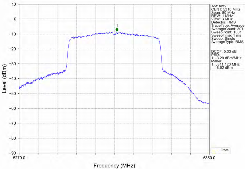
802.11ax(HEW40)_HCH_5310MHz_RU484_Left_Ant2_NTNV
