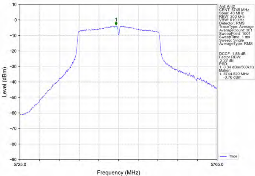
802.11a_LCH_5745MHz_Ant2_NTNV
