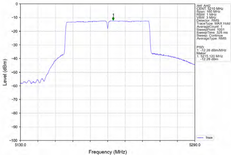
802.11ac(VHT80)_MCH_5210MHz_Ant2_NTNV
