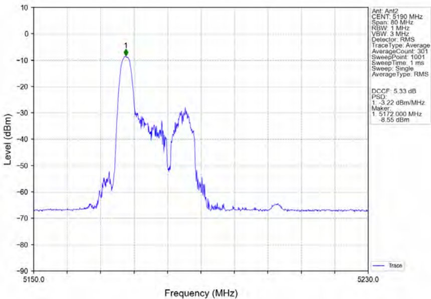
802.11ax(HEW40)_LCH_5190MHz_RU26_Left_Ant2_NTNV
