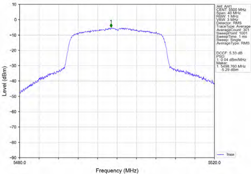
802.11ax(HEW20)_LCH_5500MHz_RU242_Left_Ant1_NTNV
