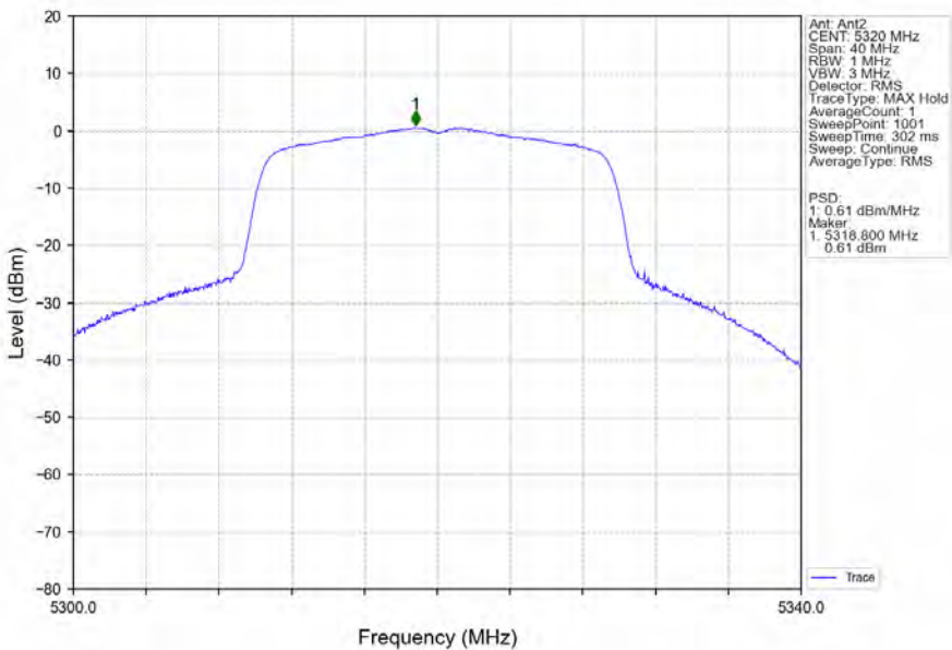
802.11ax(HEW20)_HCH_5320MHz_RU242_Left_Ant2_NTNV
