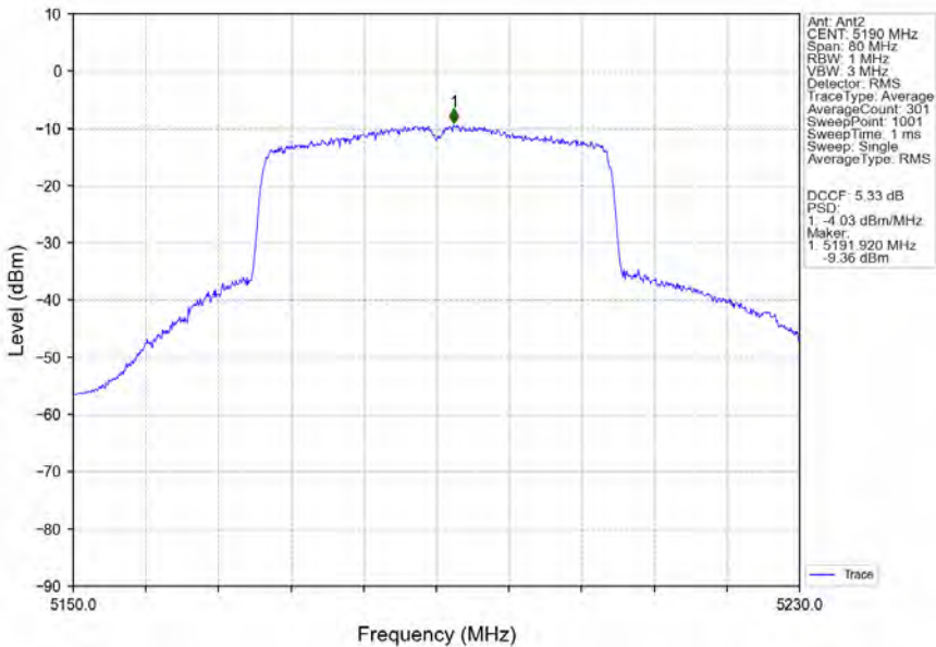
802.11ax(HEW40)_LCH_5190MHz_RU484_Left_Ant2_NTNV
