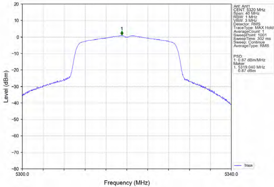
802.11ax(HEW20)_HCH_5320MHz_RU242_Left_Ant1_NTNV
