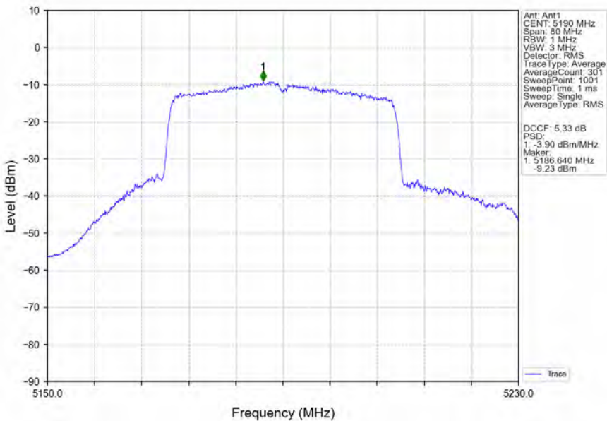
802.11ax(HEW40)_LCH_5190MHz_RU484_Left_Ant1_NTNV
