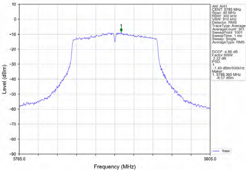
802.11n(HT20)_MCH_5785MHz_Ant1_NTNV
