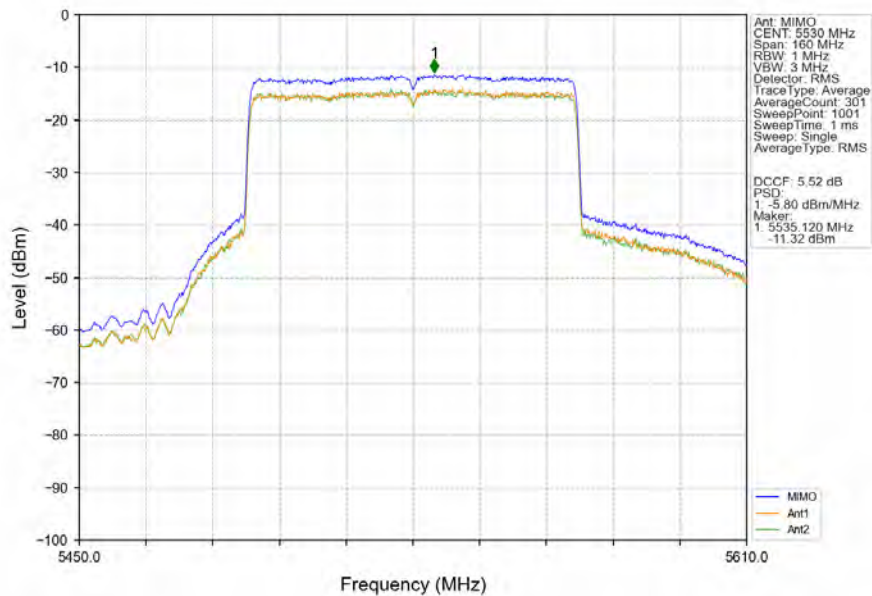
802.11ax(HEW80)_LCH_5530MHz_RU996_Left_MIMO_NTNV
