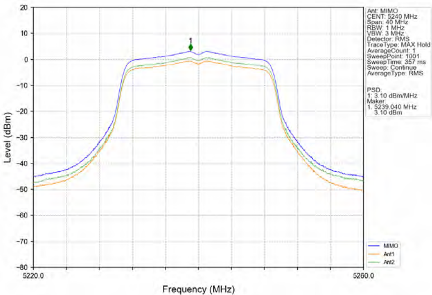
802.11n(HT20)_HCH_5240MHz_MIMO_NTNV
