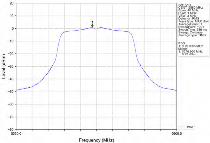
802.11n(HT20)_MCH_5580MHz_Ant1_NTNV
