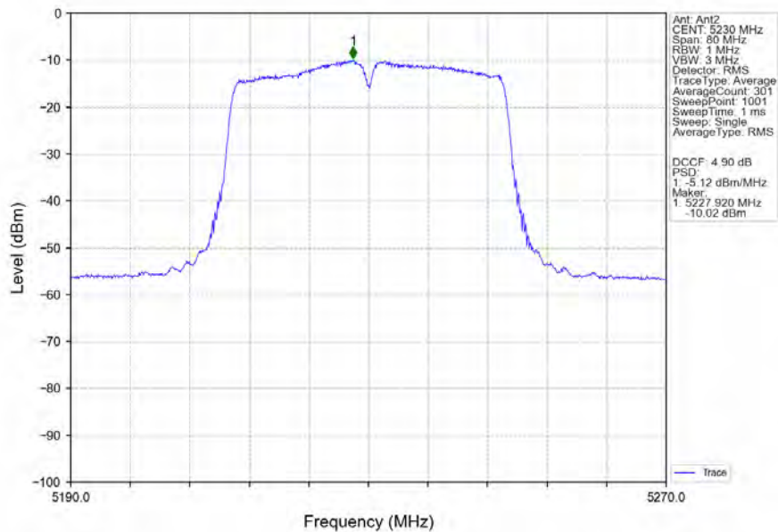
802.11n(HT40)_HCH_5230MHz_Ant2_NTNV
