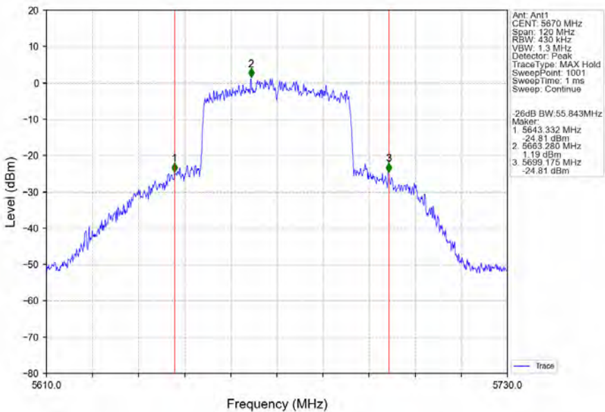
802.11ax(HEW40)_HCH_5670MHz_RU484_Left_Ant1_NTNV
