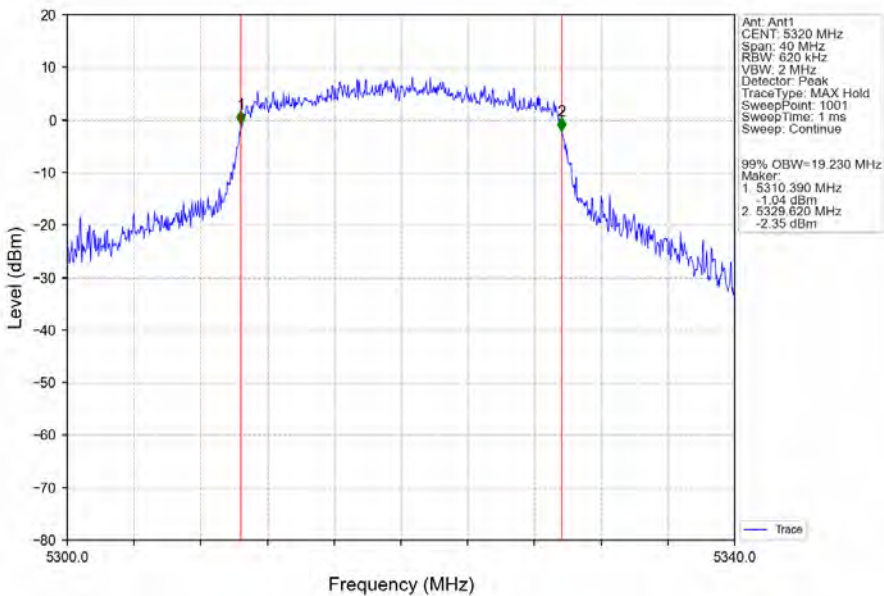
802.11ax(HEW20)_HCH_5320MHz_RU242_Left_Ant1_NTNV
