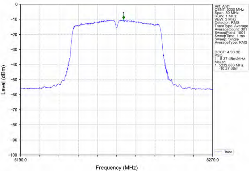
802.11n(HT40)_HCH_5230MHz_Ant1_NTNV
