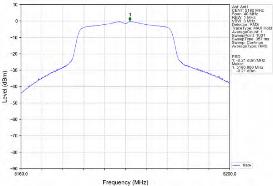
802.11n(HT20)_LCH_5180MHz_Ant1_NTNV
