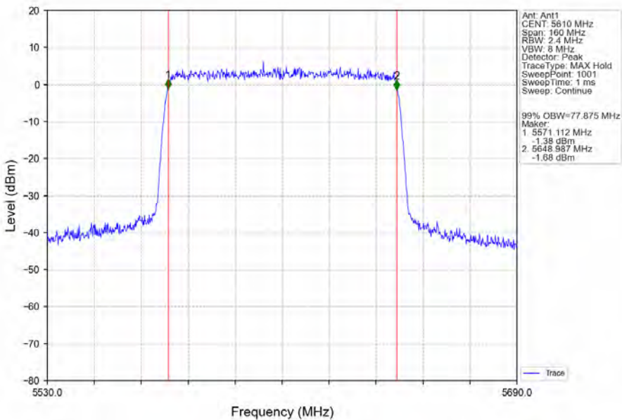
802.11ax(HEW80)_HCH_5610MHz_RU996_Left_Ant1_NTNV
