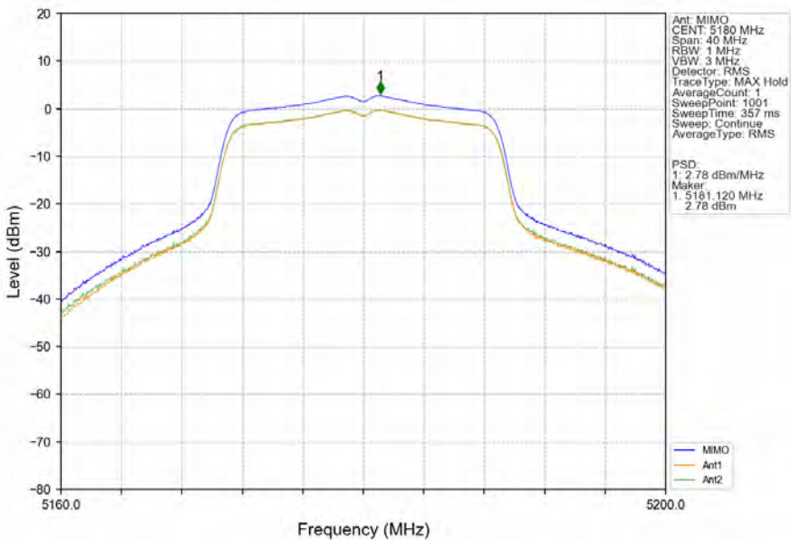
802.11n(HT20)_LCH_5180MHz_MIMO_NTNV
