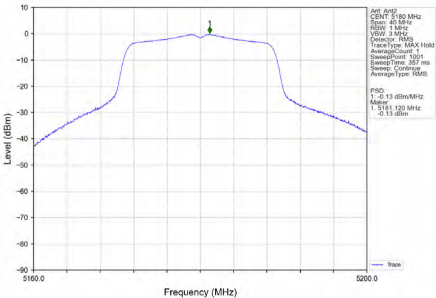
802.11n(HT20)_LCH_5180MHz_Ant2_NTNV
