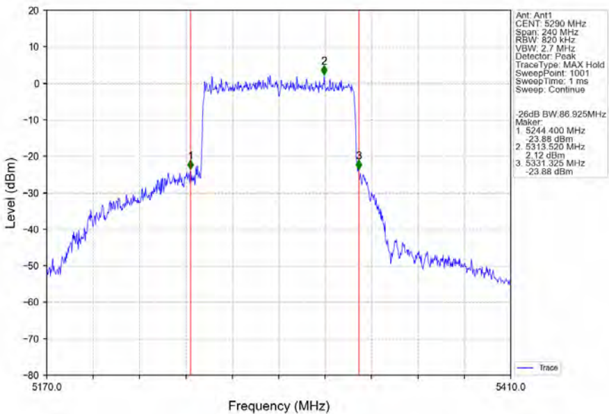
802.11ax(HEW80)_MCH_5290MHz_RU996_Left_Ant1_NTNV
