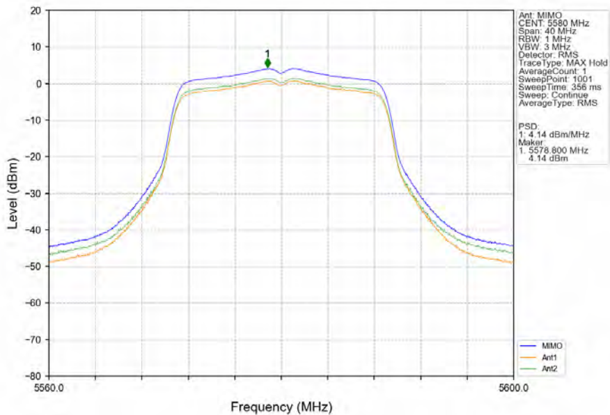
802.11n(HT20)_MCH_5580MHz_MIMO_NTNV
