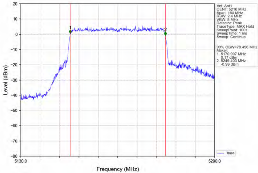
802.11ax(HEW80)_MCH_5210MHz_RU996_Left_Ant1_NTNV
