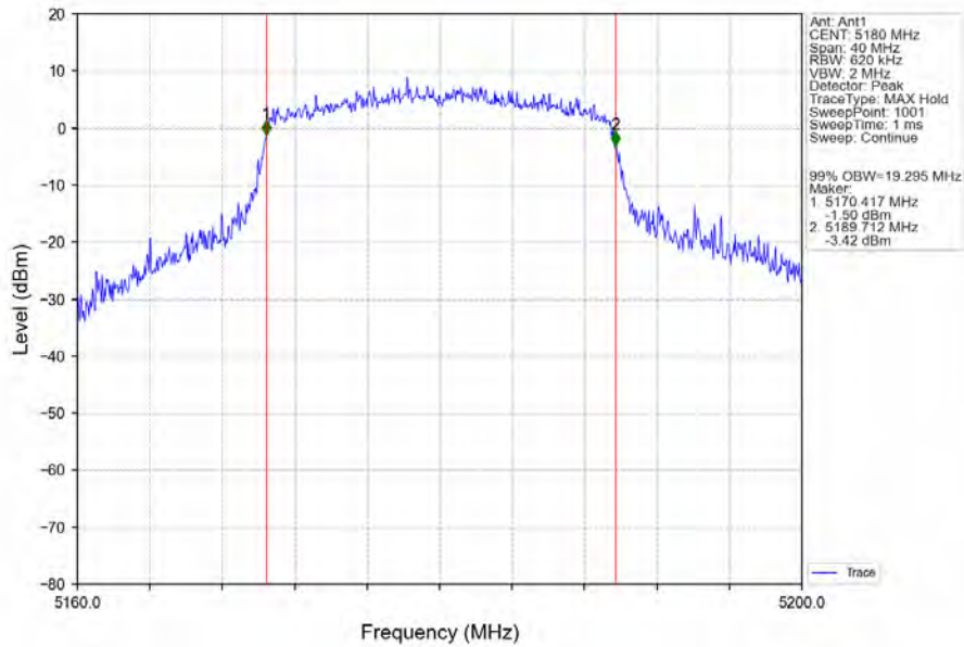
802.11ax(HEW20)_LCH_5180MHz_RU242_Left_Ant1_NTNV
