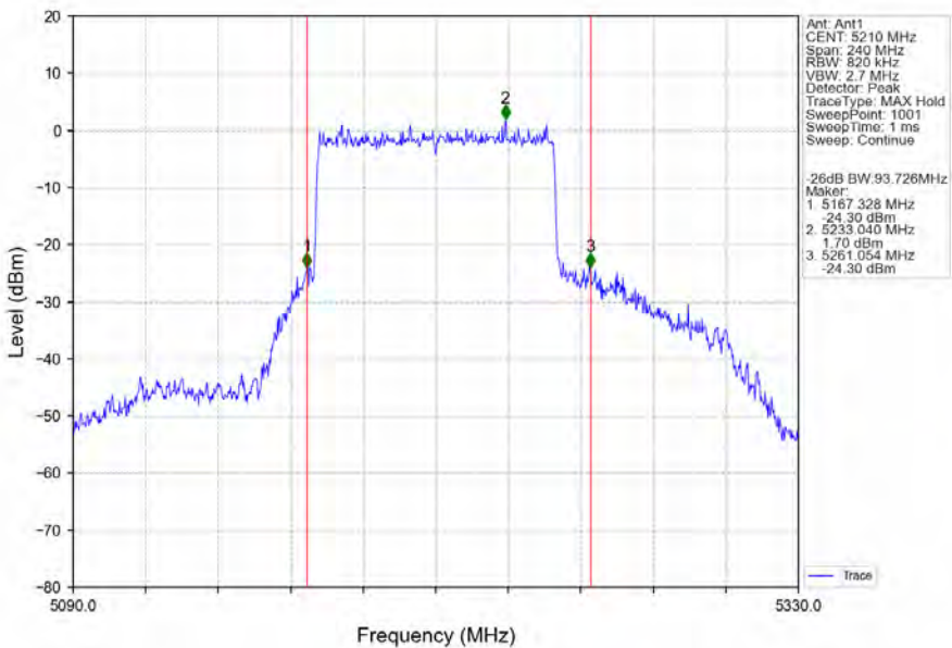
802.11ax(HEW80)_MCH_5210MHz_RU996_Left_Ant1_NTNV
