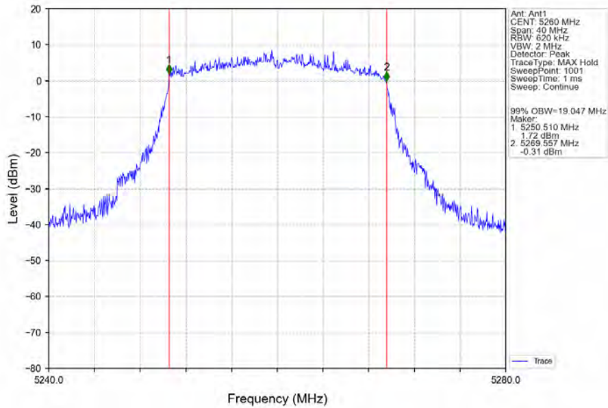
802.11ax(HEW20)_LCH_5260MHz_RU242_Left_Ant1_NTNV
