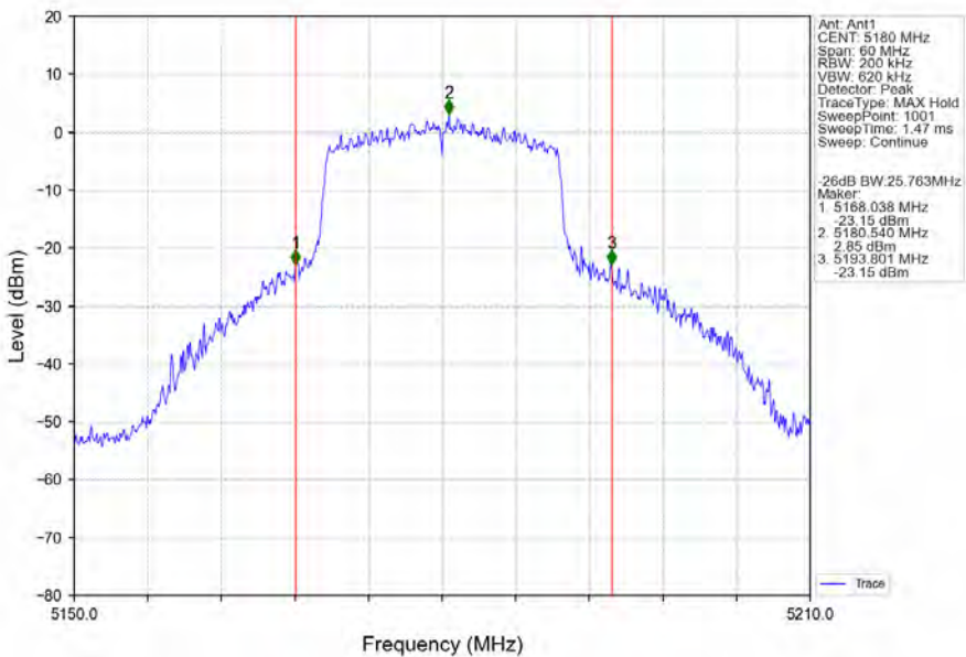
802.11ax(HEW20)_LCH_5180MHz_RU242_Left_Ant1_NTNV
