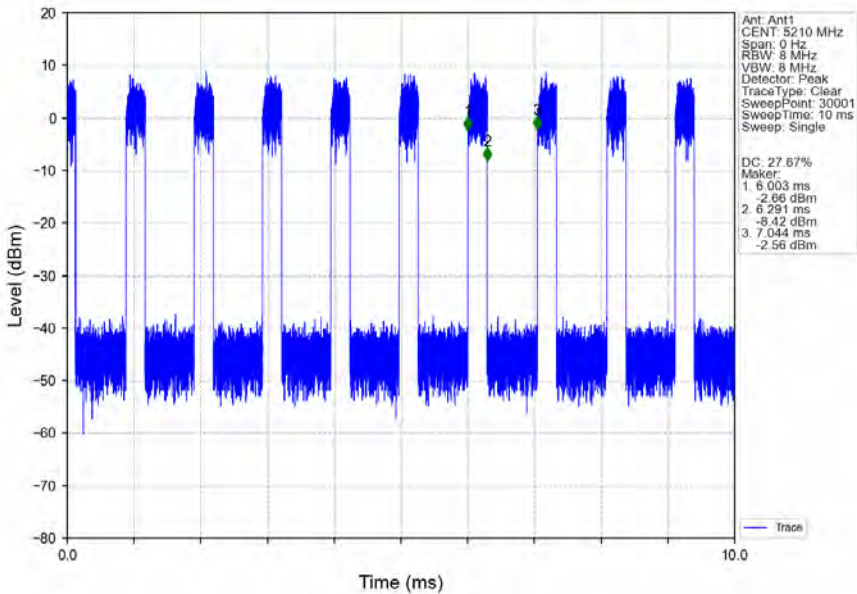
802.11ax(HEW80)_MCH_5210MHz_RU996_Left_Ant1_NTNV
