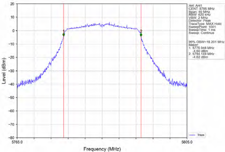
802.11n(HT20)_MCH_5785MHz_Ant1_NTNV
