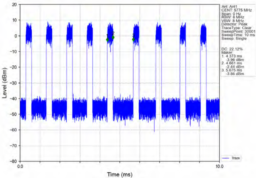
802.11ax(HEW80)_MCH_5775MHz_RU996_Left_Ant1_NTNV
