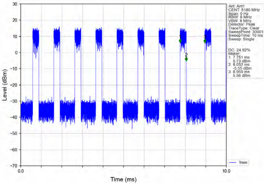
802.11ax(HEW20)_LCH_5180MHz_RU242_Left_Ant1_NTNV
