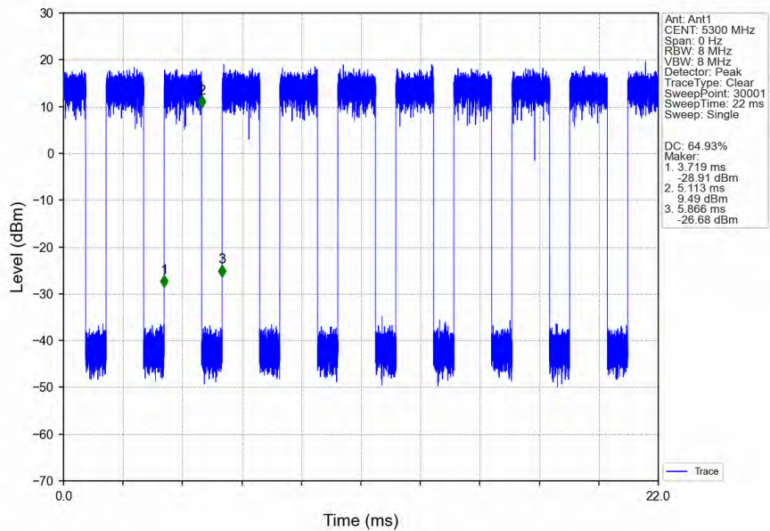
802.11a_MCH_5300MHz_Ant1_NTNV
