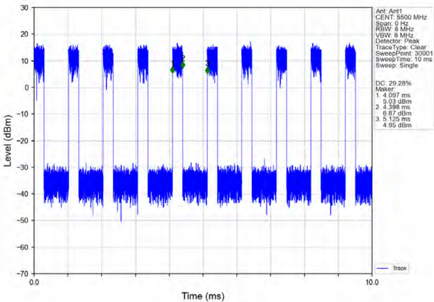
802.11ax(HEW20)_LCH_5500MHz_RU242_Left_Ant1_NTNV
