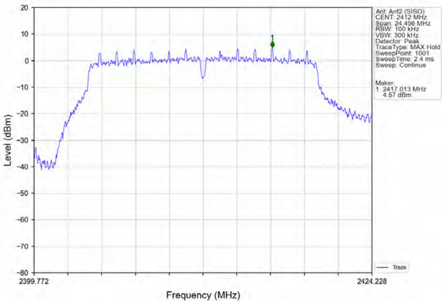
802.11g_LCH_2412MHz_Ant2 (SISO)_NTNV
