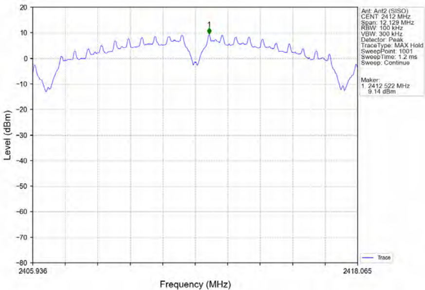
802.11b_LCH_2412MHz_Ant2 (SISO)_NTNV
