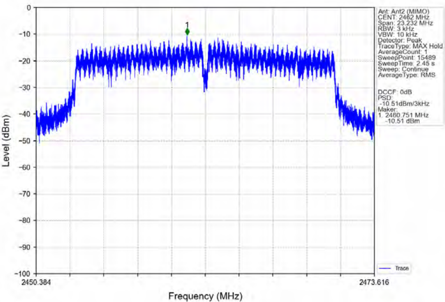
802.11n(HT20)_HCH_2462MHz_Ant2 (MIMO)_NTNV
