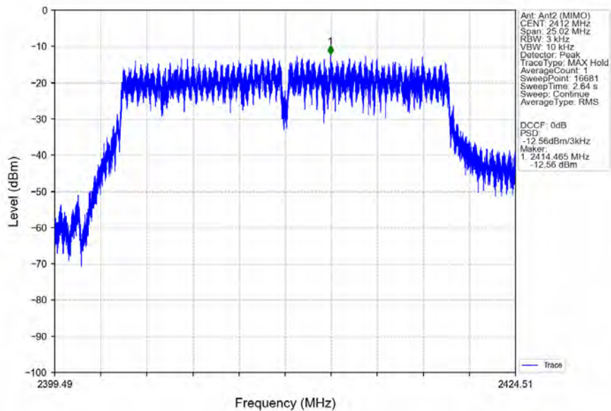
802.11n(HT20)_LCH_2412MHz_Ant2 (MIMO)_NTNV
