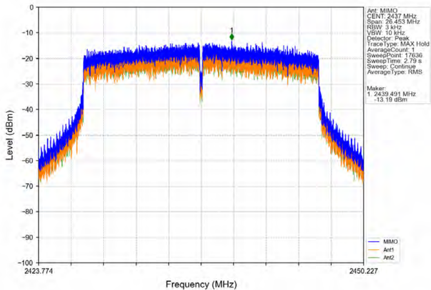
802.11ax(HEW20)_MCH_2437MHz_RU242_Left_MIMO_NTNV
