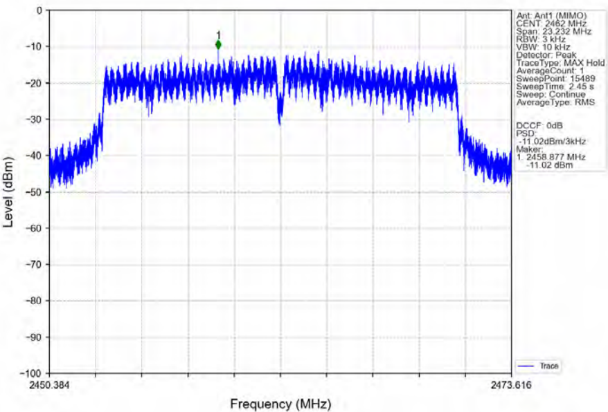
802.11n(HT20)_HCH_2462MHz_Ant1 (MIMO)_NTNV
