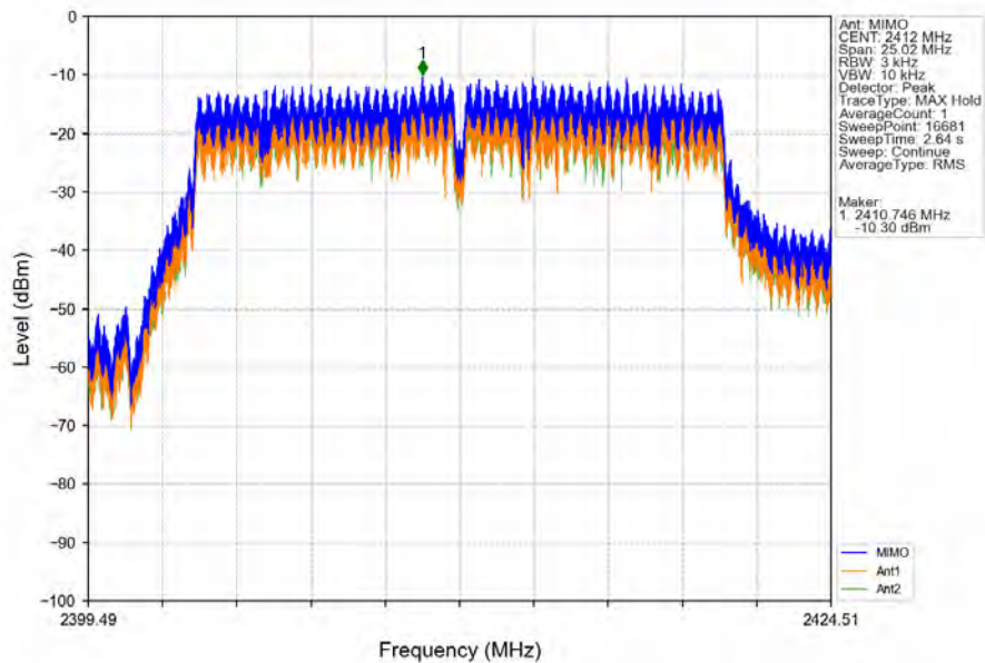
802.11n(HT20)_LCH_2412MHz_MIMO_NTNV
