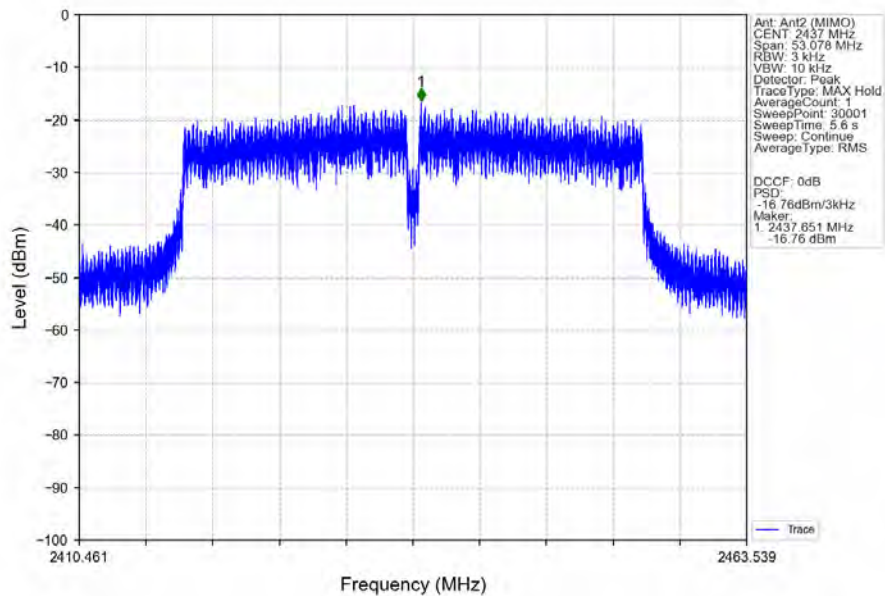
802.11n(HT40)_MCH_2437MHz_Ant2 (MIMO)_NTNV
