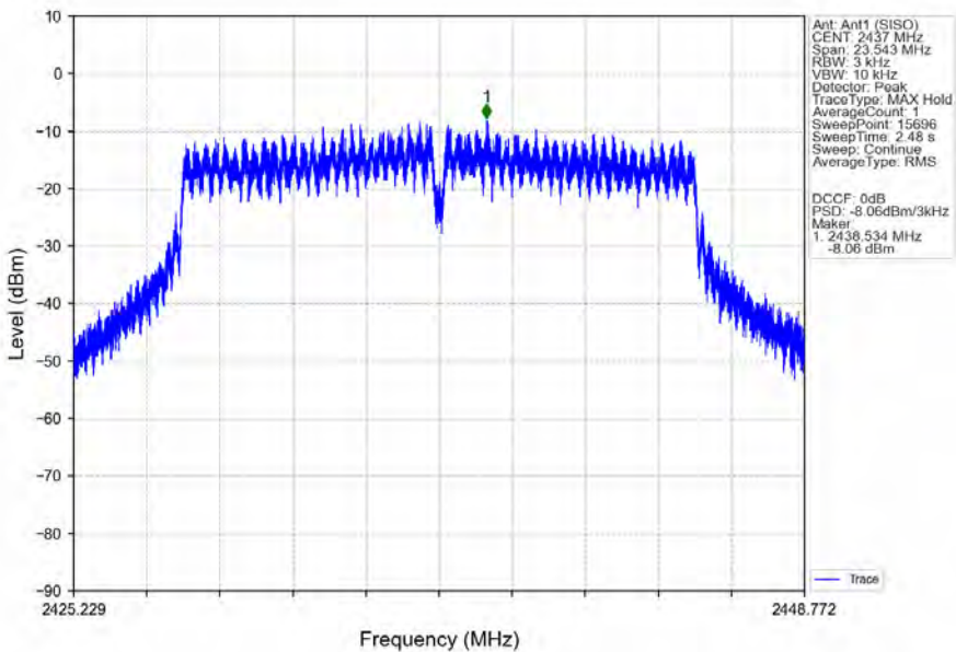
802.11g_MCH_2437MHz_Ant1 (SISO)_NTNV
