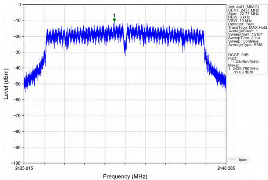
802.11n(HT20)_MCH_2437MHz_Ant1 (MIMO)_NTNV
