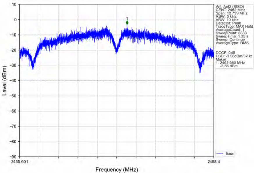
802.11b_HCH_2462MHz_Ant2 (SISO)_NTNV
