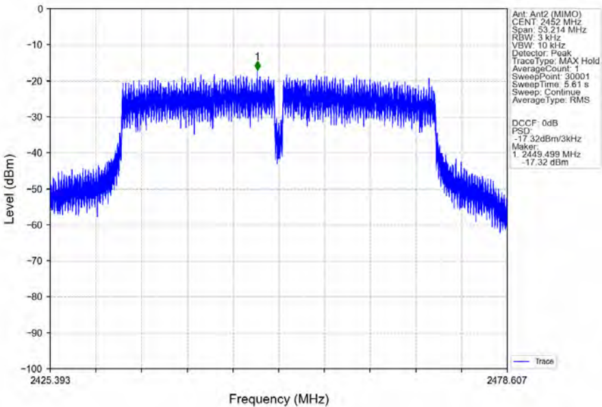
802.11n(HT40)_HCH_2452MHz_Ant2 (MIMO)_NTNV
