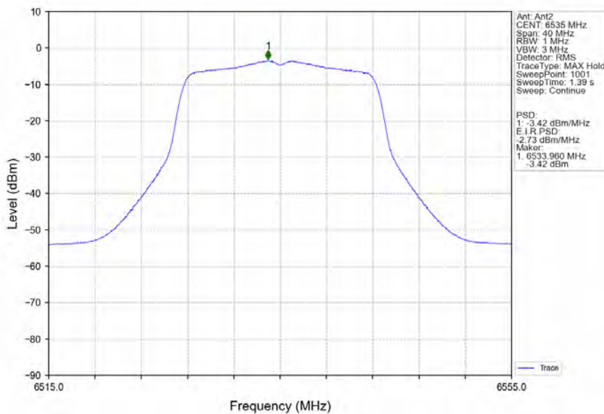
802.11a_LCH_6535MHz_Ant2_NTNV
