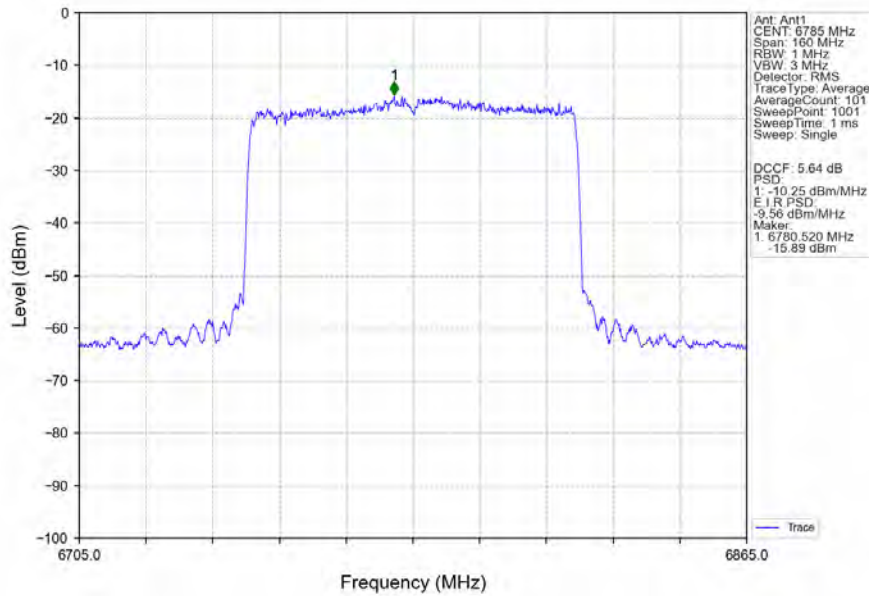
802.11ax(HEW80)_HCH_6785MHz_RU996_Left_Ant1_NTNV
