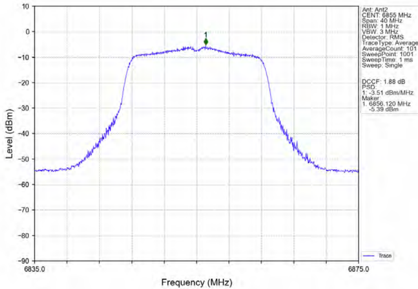
802.11a_HCH_6855MHz_Ant2_NTNV
