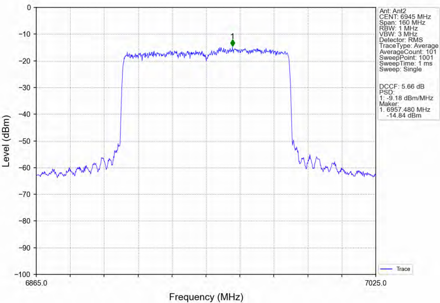
802.11ax(HEW80)_LCH_6945MHz_RU996_Left_Ant2_NTNV
