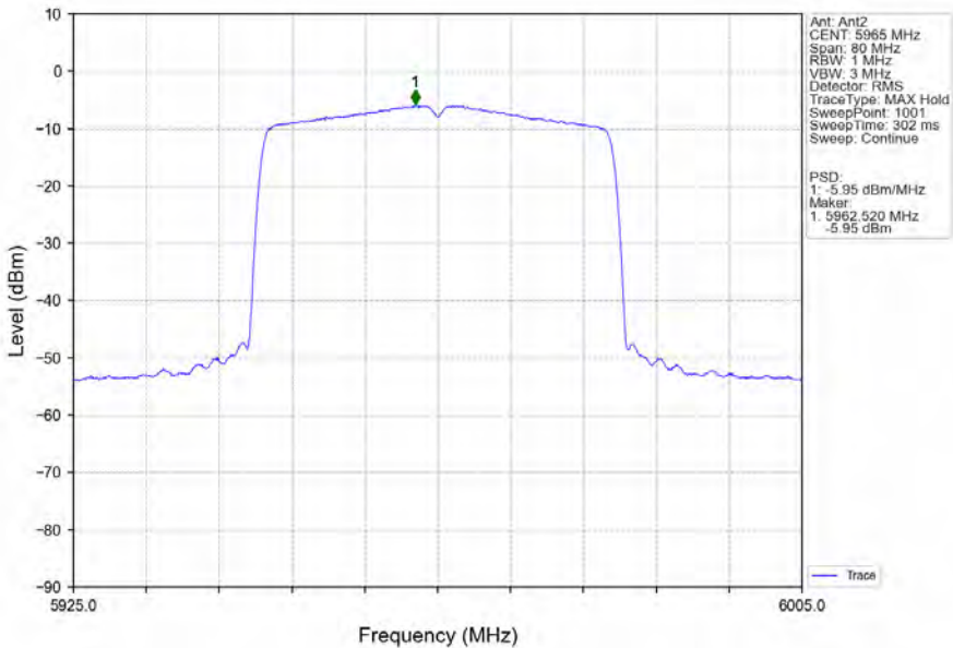
802.11ax(HEW40)_LCH_5965MHz_RU484_Left_Ant2_NTNV
