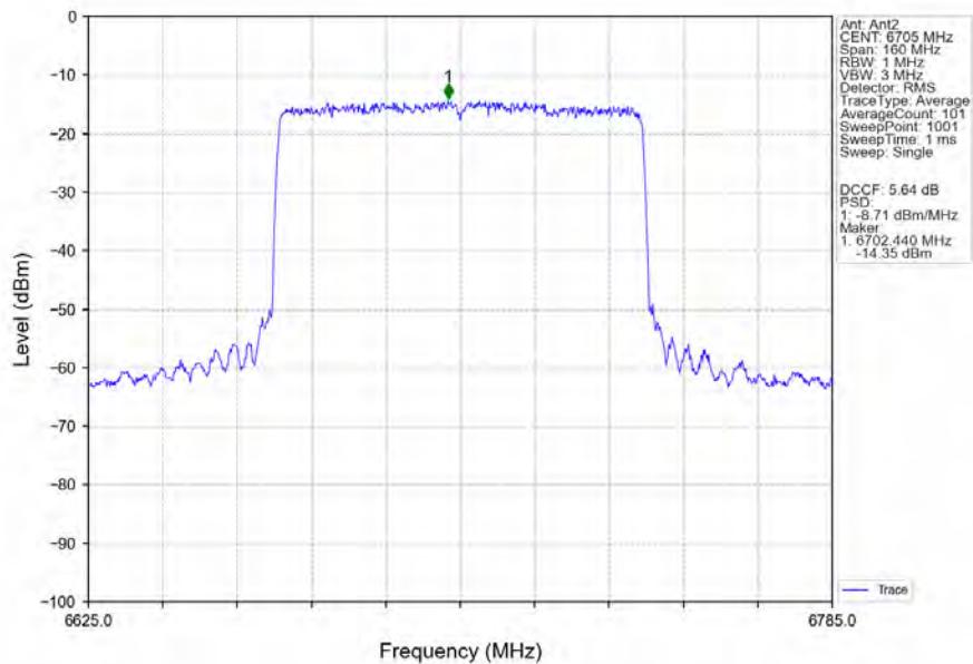
802.11ax(HEW80)_MCH_6705MHz_RU996_Left_Ant2_NTNV
