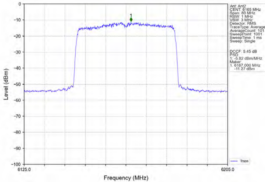
802.11ax(HEW40)_MCH_6165MHz_RU484_Left_Ant2_NTNV
