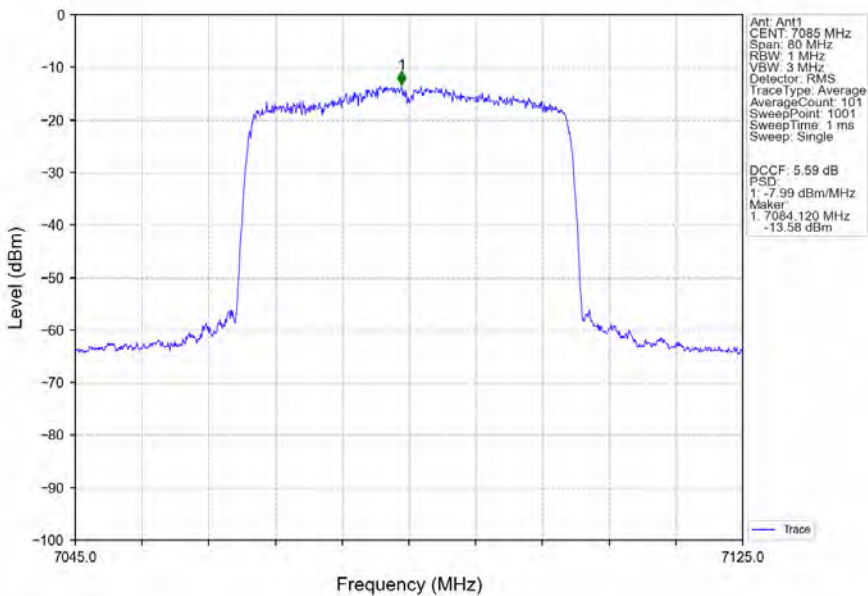
802.11ax(HEW40)_HCH_7085MHz_RU484_Left_Ant1_NTNV
