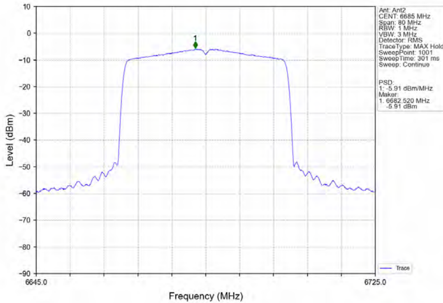
802.11ax(HEW40)_MCH_6685MHz_RU484_Left_Ant2_NTNV
