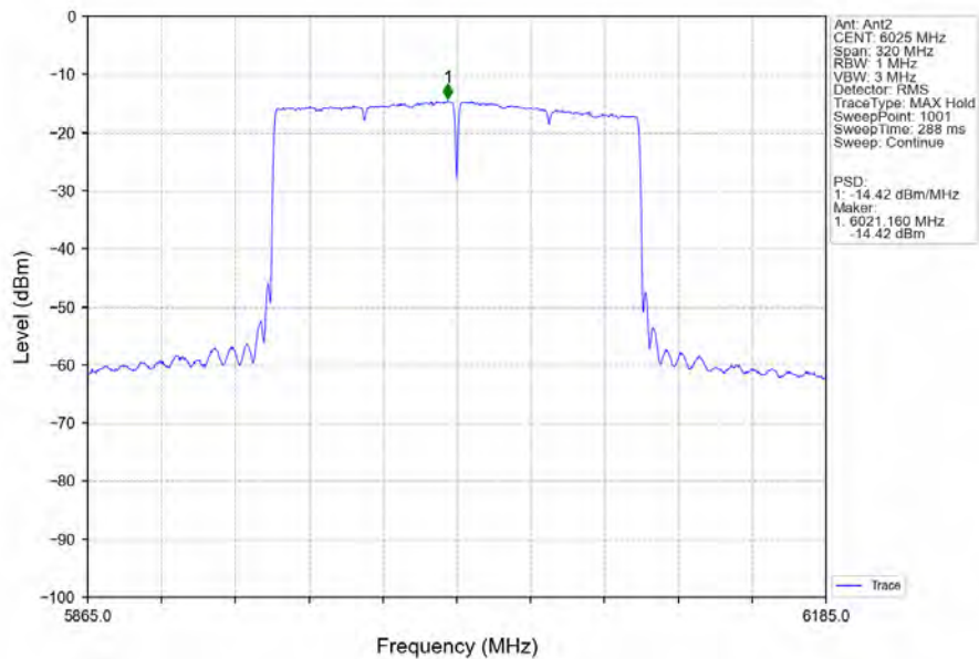
802.11ax(HEW160)_LCH_6025MHz_2xRU996_Left_Ant2_NTNV
