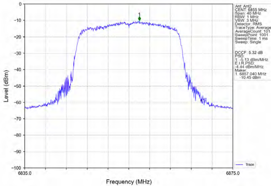
802.11ax(HEW20)_HCH_6855MHz_RU242_Left_Ant2_NTNV
