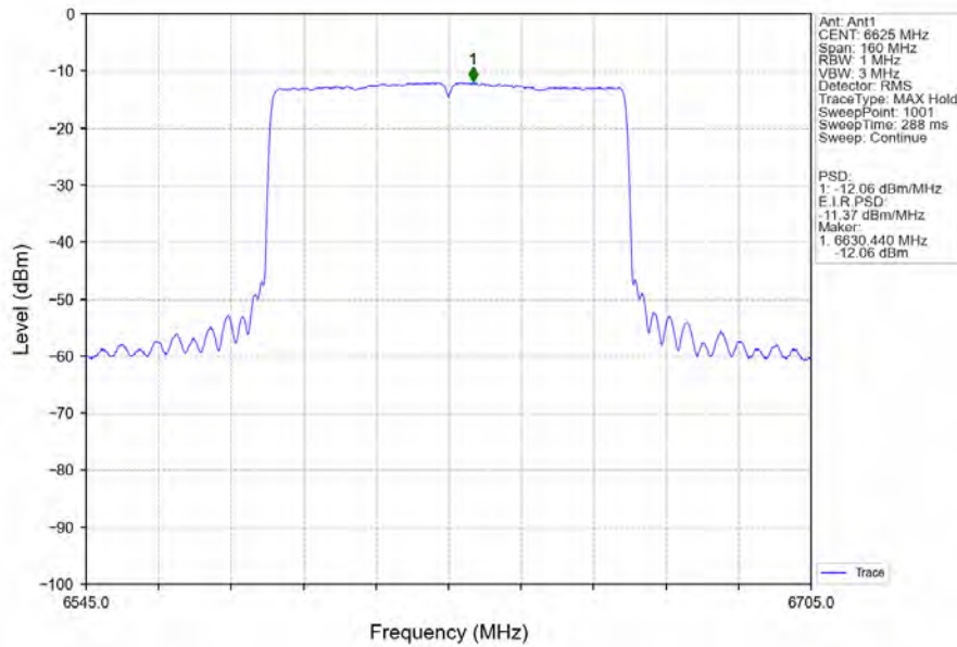
802.11ax(HEW80)_LCH_6625MHz_RU996_Left_Ant1_NTNV
