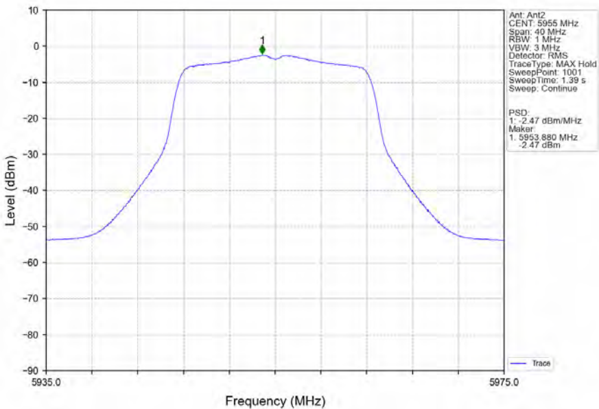
802.11a_LCH_5955MHz_Ant2_NTNV
