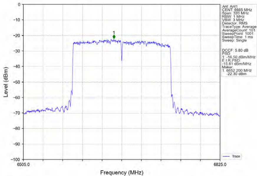
802.11ax(HEW160)_MCH_6665MHz_2xRU996_Left_Ant1_NTNV
