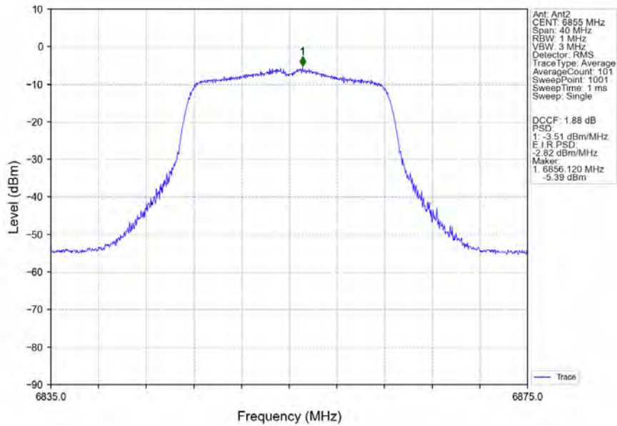
802.11a_HCH_6855MHz_Ant2_NTNV
