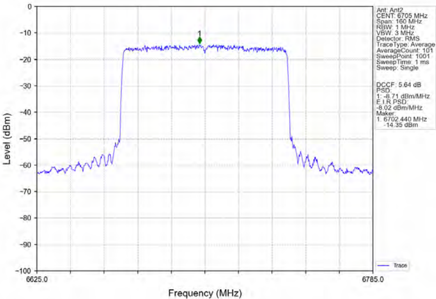
802.11ax(HEW80)_MCH_6705MHz_RU996_Left_Ant2_NTNV
