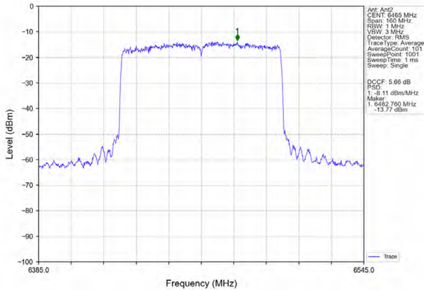
802.11ax(HEW80)_LCH_6465MHz_RU996_Left_Ant2_NTNV
