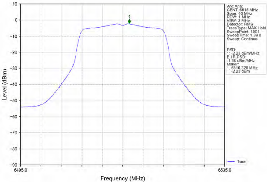
802.11a_HCH_6515MHz_Ant2_NTNV
