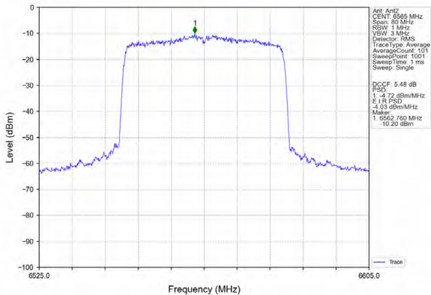
802.11ax(HEW40)_LCH_6565MHz_RU484_Left_Ant2_NTNV
