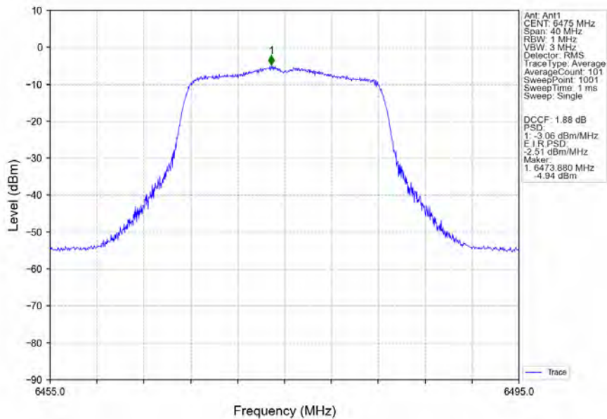
802.11a_MCH_6475MHz_Ant1_NTNV
