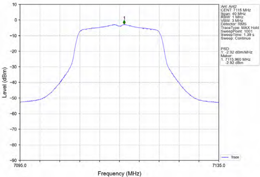
802.11a_HCH_7115MHz_Ant2_NTNV
