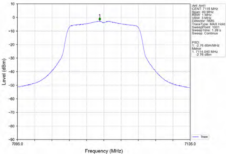
802.11a_HCH_7115MHz_Ant1_NTNV
