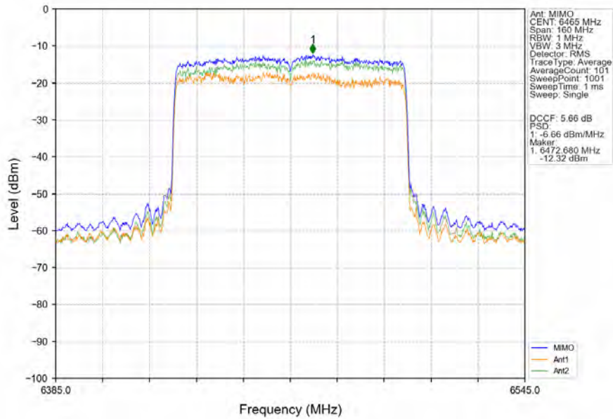
802.11ax(HEW80)_LCH_6465MHz_RU996_Left_MIMO_NTNV
