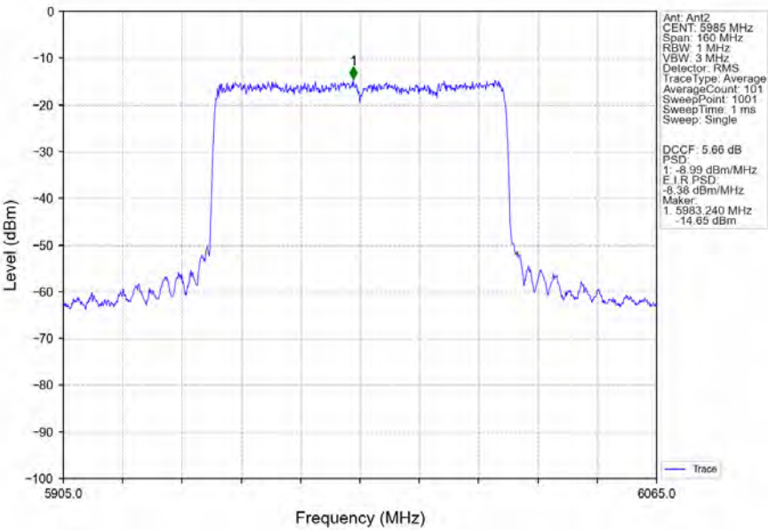
802.11ax(HEW80)_LCH_5985MHz_RU996_Left_Ant2_NTNV
