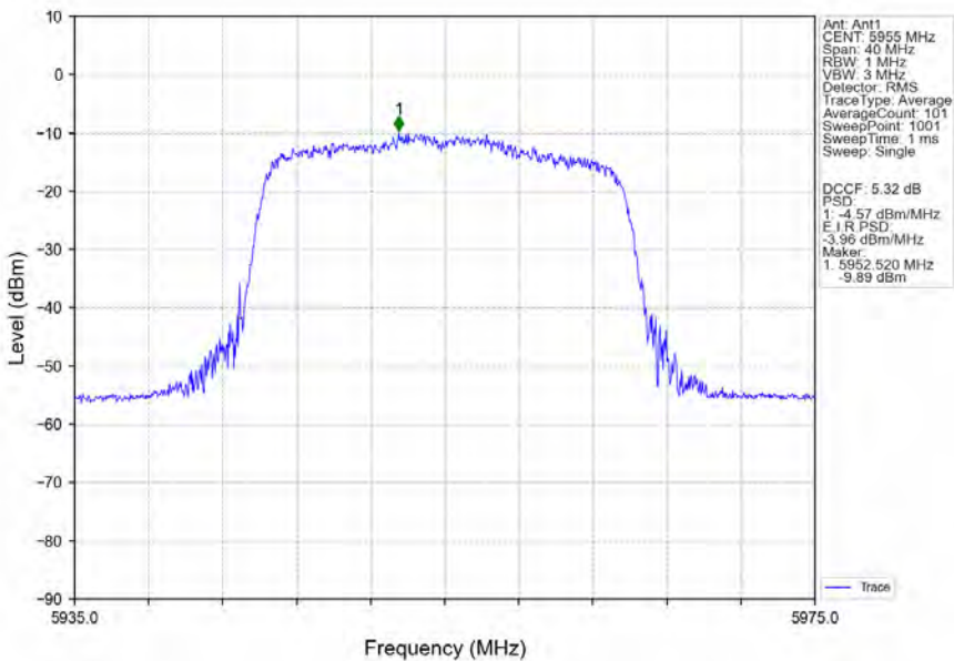
802.11ax(HEW20)_LCH_5955MHz_RU242_Left_Ant1_NTNV
