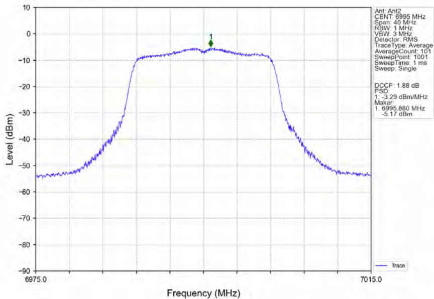
802.11a_MCH_6995MHz_Ant2_NTNV
