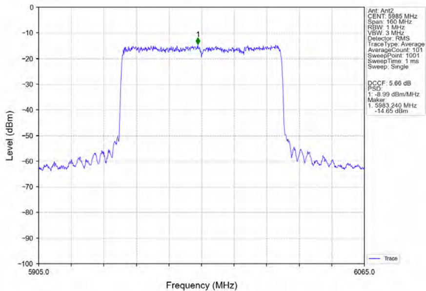
802.11ax(HEW80)_LCH_5985MHz_RU996_Left_Ant2_NTNV
