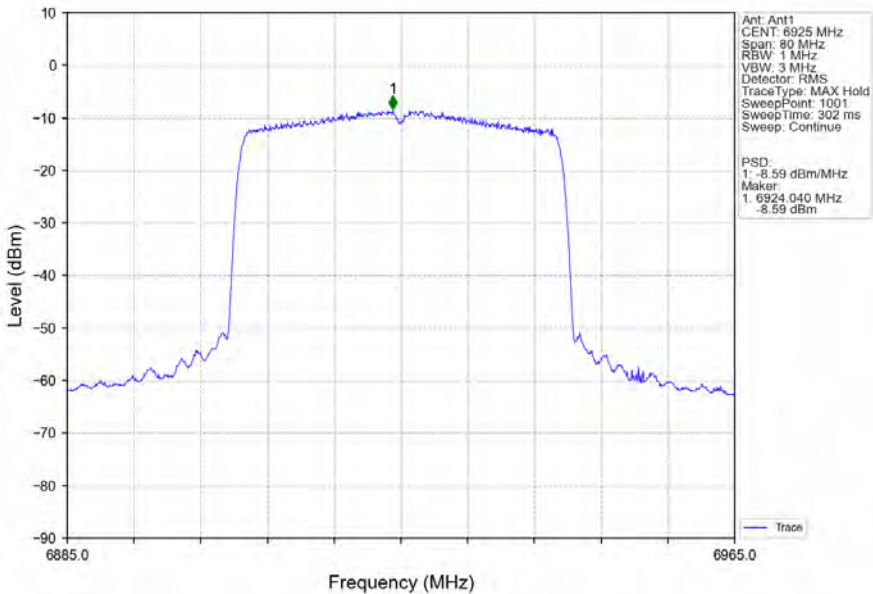
802.11ax(HEW40)_LCH_6925MHz_RU484_Left_Ant1_NTNV
