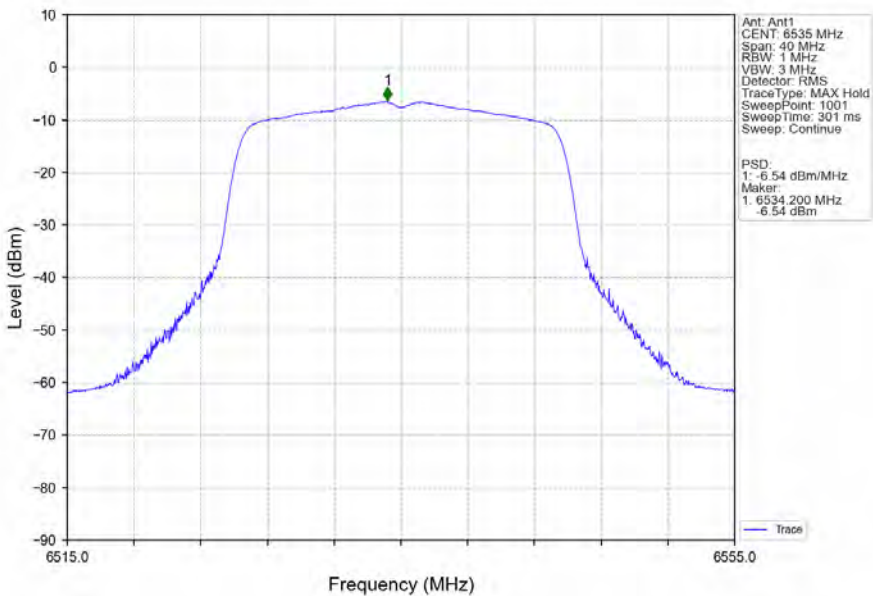
802.11ax(HEW20)_LCH_6535MHz_RU242_Left_Ant1_NTNV
