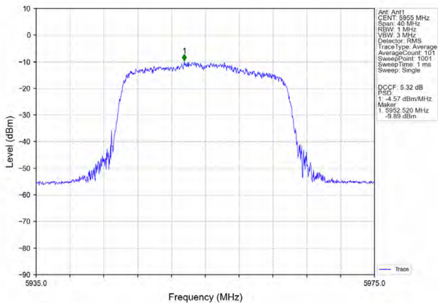
802.11ax(HEW20)_LCH_5955MHz_RU242_Left_Ant1_NTNV
