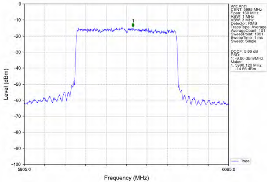
802.11ax(HEW80)_LCH_5985MHz_RU996_Left_Ant1_NTNV
