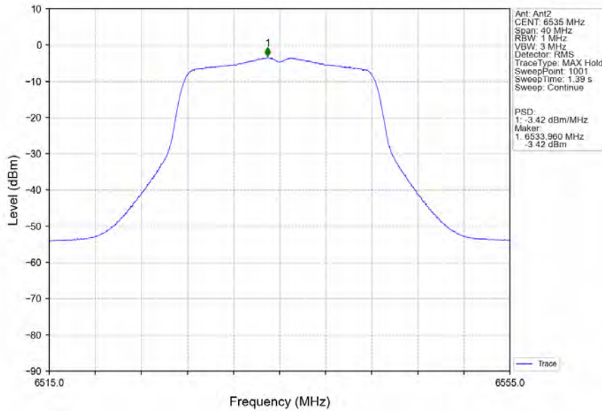
802.11a_LCH_6535MHz_Ant2_NTNV
