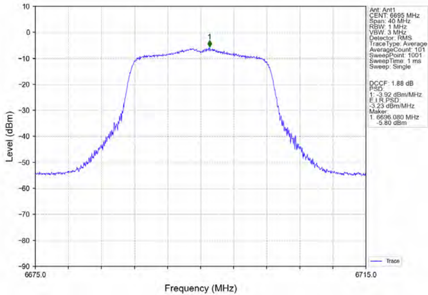
802.11a_MCH_6695MHz_Ant1_NTNV
