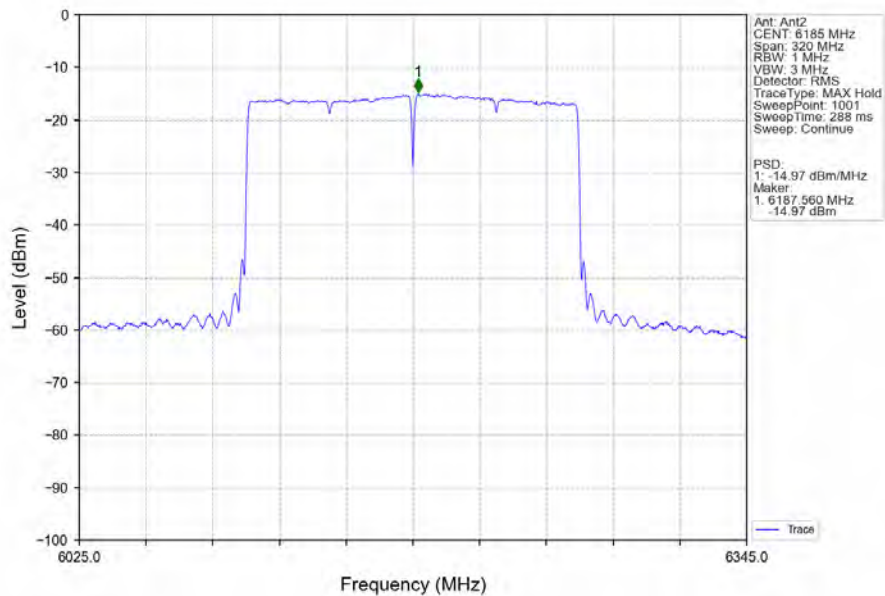
802.11ax(HEW160)_MCH_6185MHz_2xRU996_Left_Ant2_NTNV
