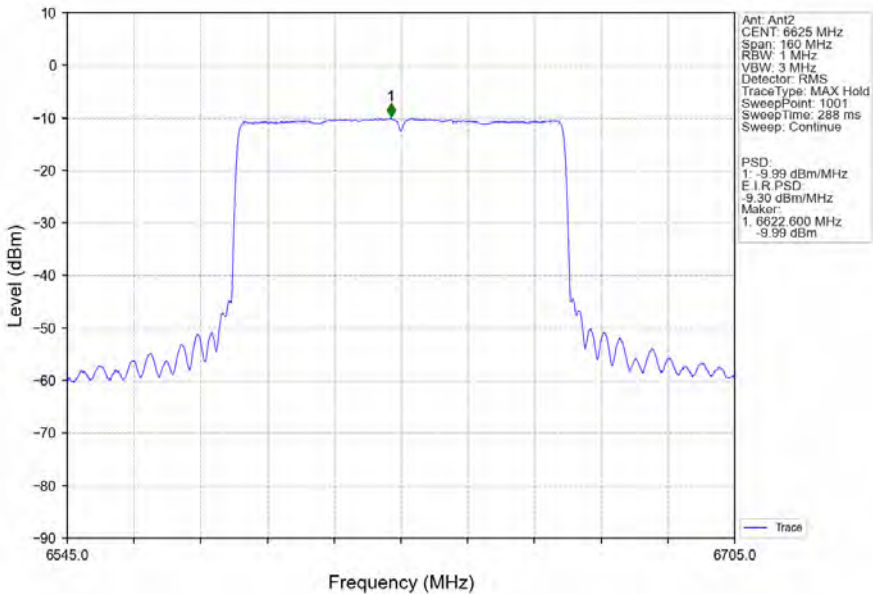
802.11ax(HEW80)_LCH_6625MHz_RU996_Left_Ant2_NTNV
