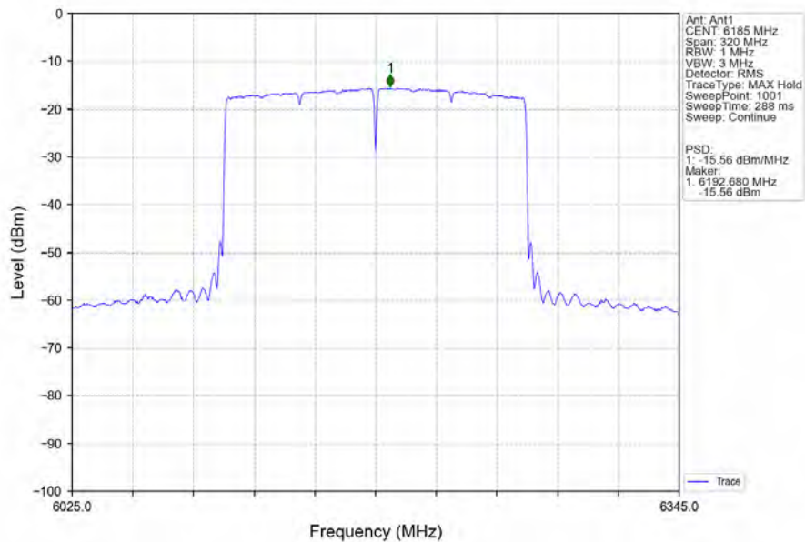
802.11ax(HEW160)_MCH_6185MHz_2xRU996_Left_Ant1_NTNV
