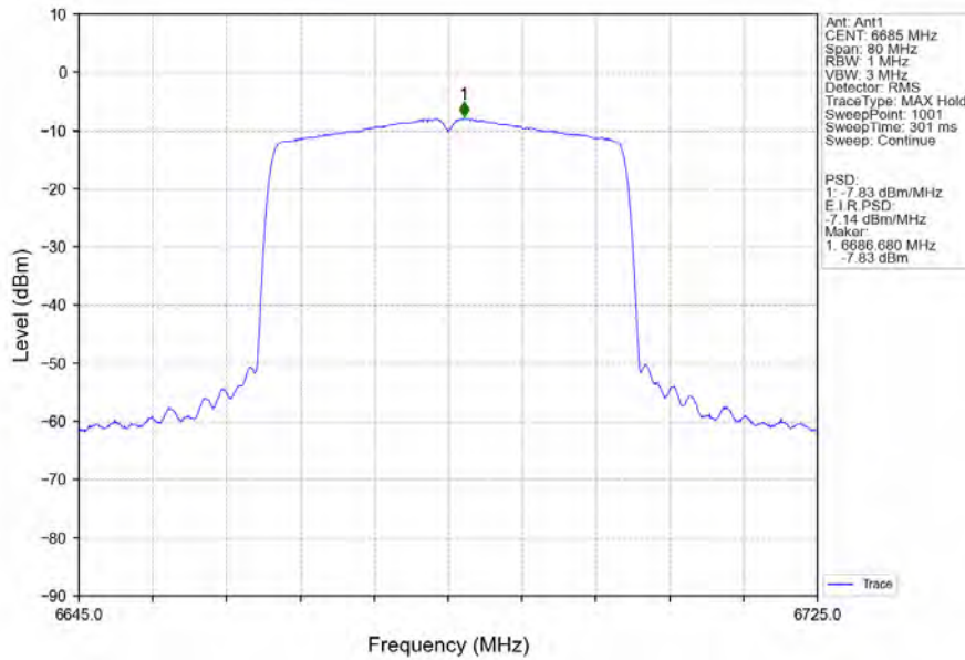
802.11ax(HEW40)_MCH_6685MHz_RU484_Left_Ant1_NTNV
