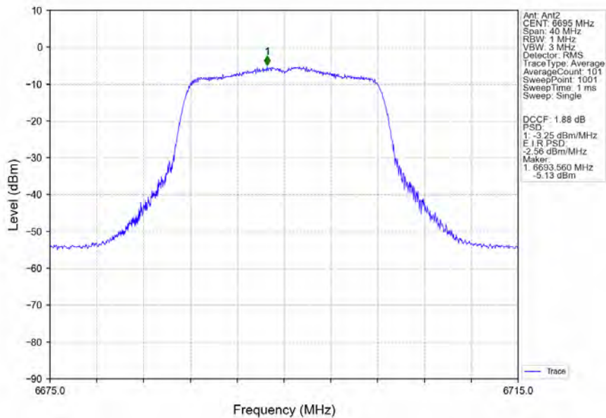
802.11a_MCH_6695MHz_Ant2_NTNV
