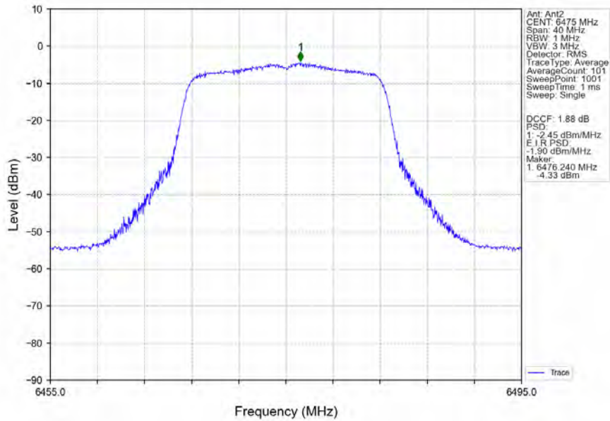
802.11a_MCH_6475MHz_Ant2_NTNV
