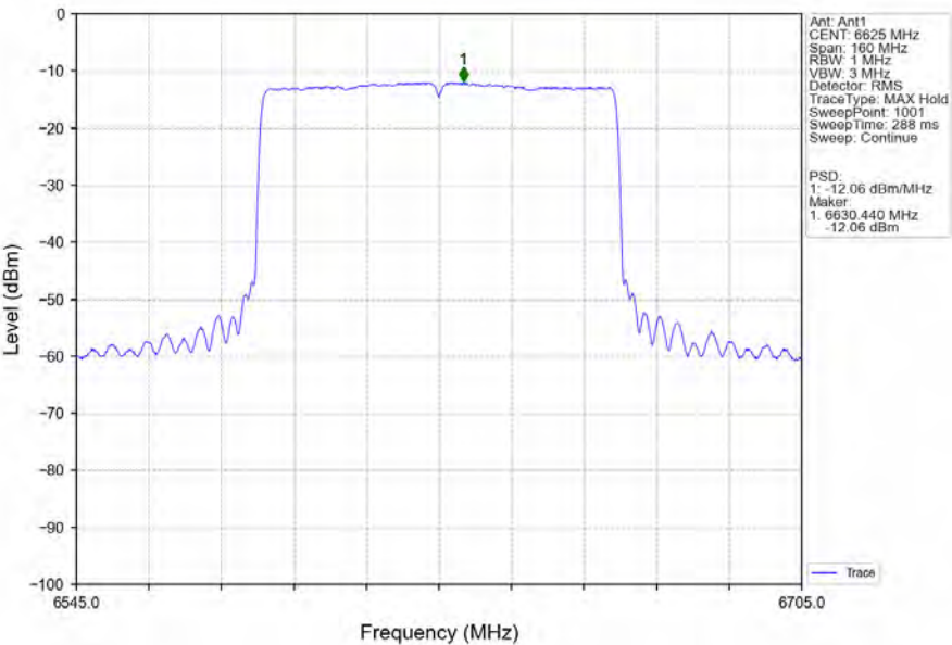
802.11ax(HEW80)_LCH_6625MHz_RU996_Left_Ant1_NTNV
