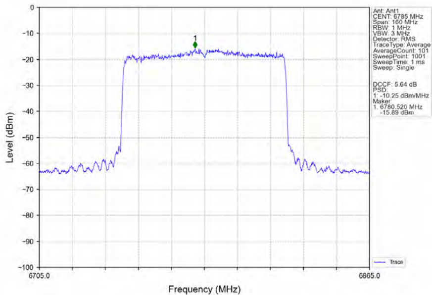
802.11ax(HEW80)_HCH_6785MHz_RU996_Left_Ant1_NTNV
