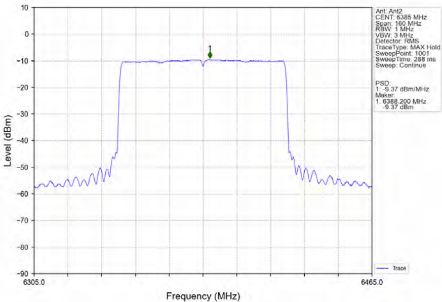
802.11ax(HEW80)_HCH_6385MHz_RU996_Left_Ant2_NTNV
