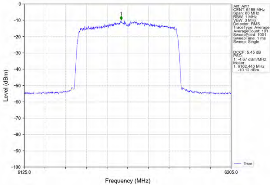
802.11ax(HEW40)_MCH_6165MHz_RU484_Left_Ant1_NTNV
