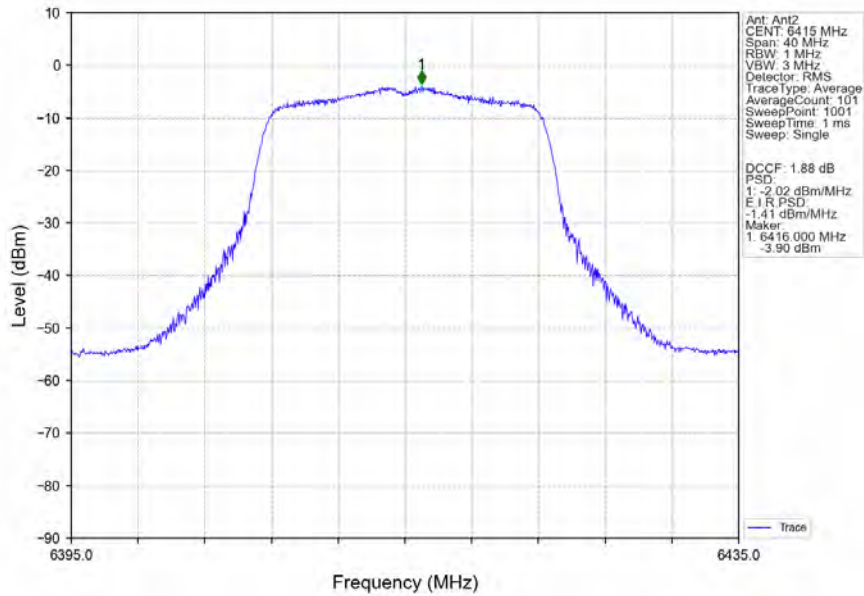
802.11a_HCH_6415MHz_Ant2_NTNV
