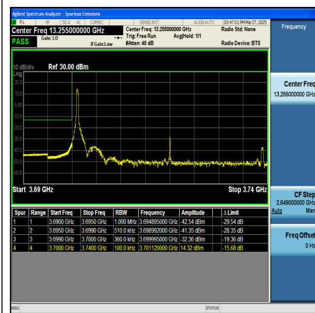
NTNV-n77(3700-3980)-PC2-30-40-L-CP-QPSK- Edge_1RB_Left-PASS
