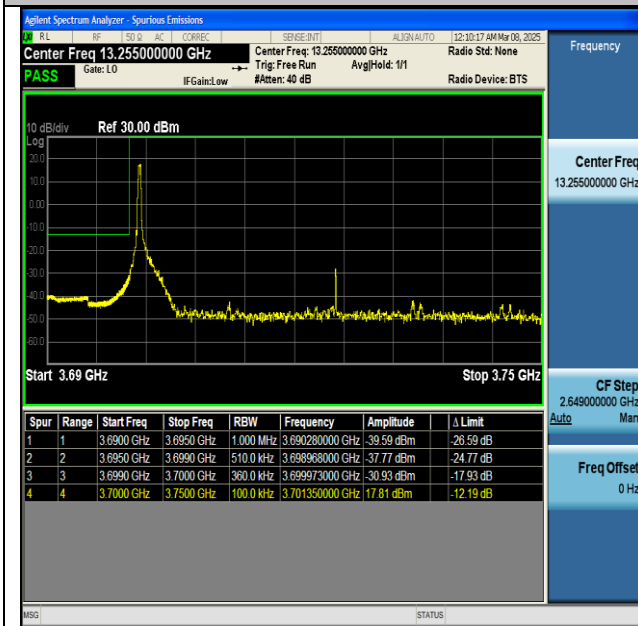
NTNV-n77(3700-3980)-PC2-30-50-L-CP-QPSK- Edge_1RB_Left-PASS
