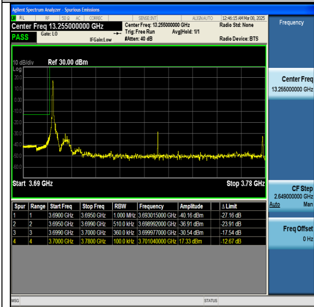
NTNV-n77(3700-3980)-PC2-30-80-L-CP-QPSK- Edge_1RB_Left-PASS
