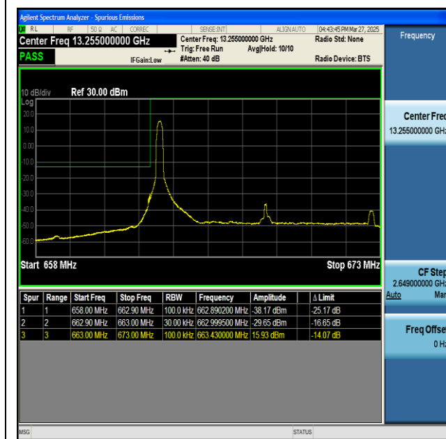
NTNV-n71-PC3-15-10-L-CP-QPSK-Edge_1RB_Left-PASS
