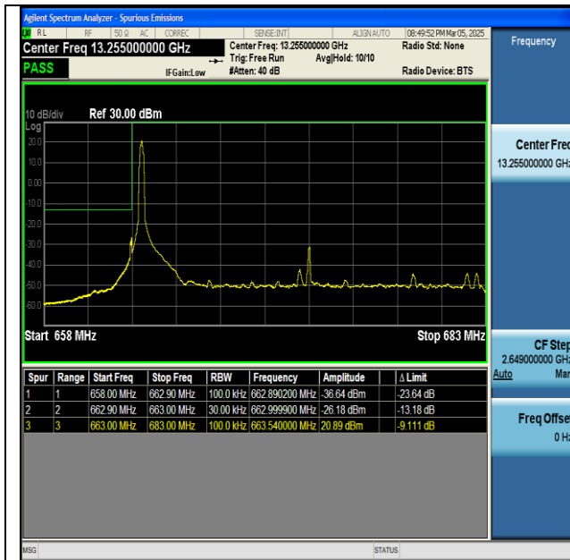
NTNV-n71-PC3-15-20-L-DFT-BPSK-Edge_1RB_Left-PASS
