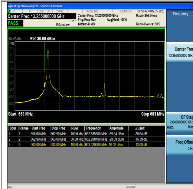
NTNV-n71-PC3-15-20-L-CP-QPSK-Edge_1RB_Left-PASS
