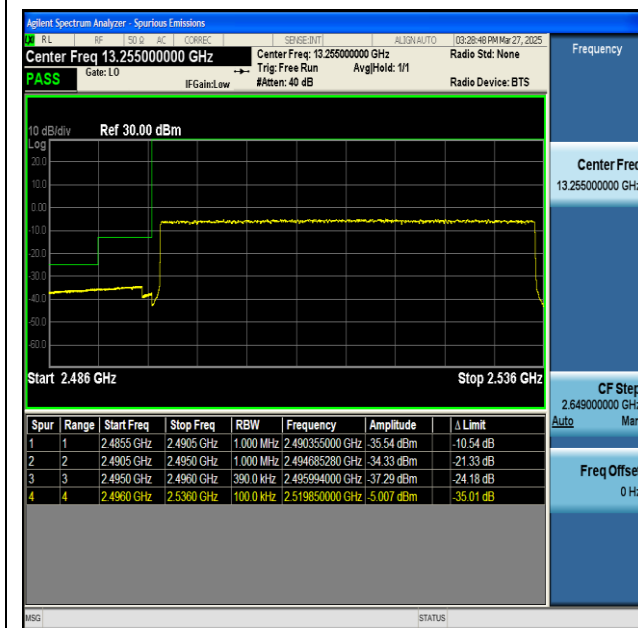
NTNV-n41-PC2-30-40-L-CP-QPSK-Edge_1RB_Left-PASS
