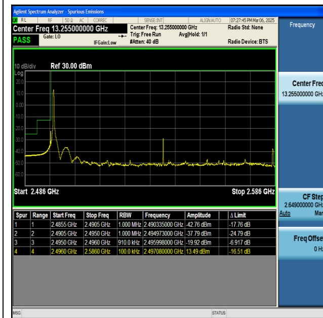
NTNV-n41-PC2-30-90-L-CP-QPSK-Edge_1RB_Left-PASS
