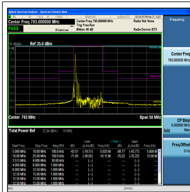
NTNT-n14-PC3-15-10-H-CP-QPSK-Inner_1RB_Left-PASS
