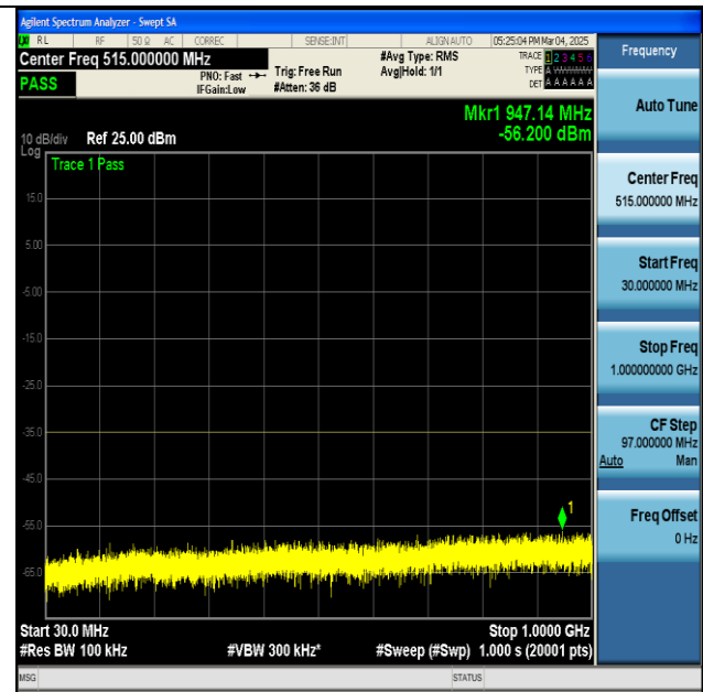
NTNV-n7-PC3-15-20-M-CP-QPSK-Edge_1RB_Left-30-1000-PASS
