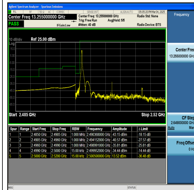
NTNV-n7-PC3-15-15-L-CP-QPSK-Edge_1RB_Left-PASS
