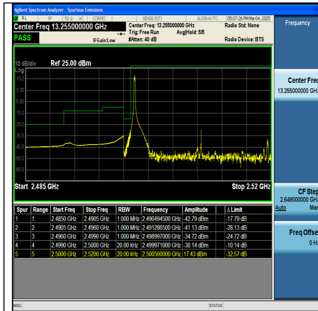
NTNV-n7-PC3-15-20-L-DFT-BPSK-Edge_1RB_Left-PASS
