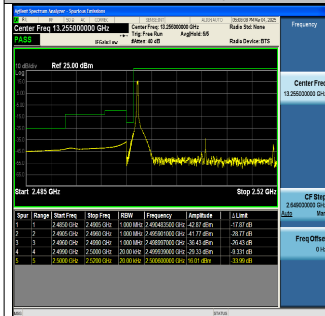
NTNV-n7-PC3-15-20-L-CP-QPSK-Edge_1RB_Left-PASS
