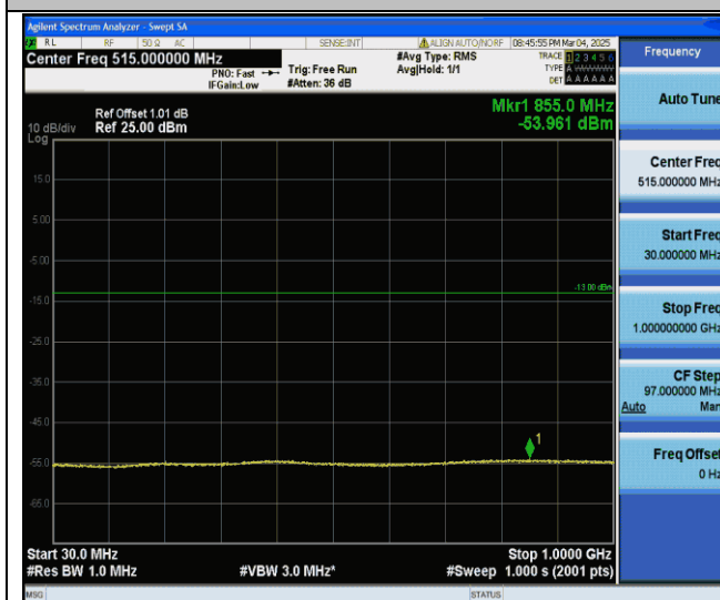
Band IV-1312-30~1000MHz-PASS
