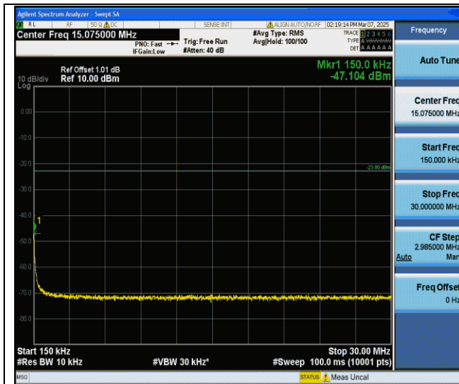
GPRS850-251-5-0.15~30MHz-PASS
