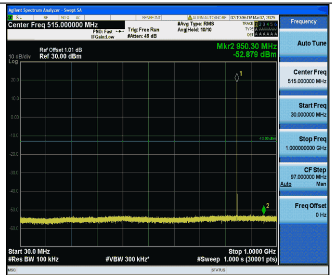
GPRS850-251-5-30~1000MHz-PASS
