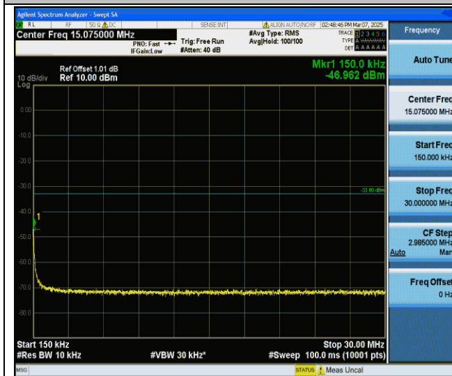
GPRS1900-512-0-0.15~30MHz-PASS
