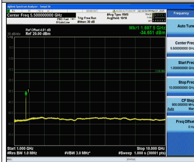
GPRS850-251-5-1000~10000MHz-PASS
