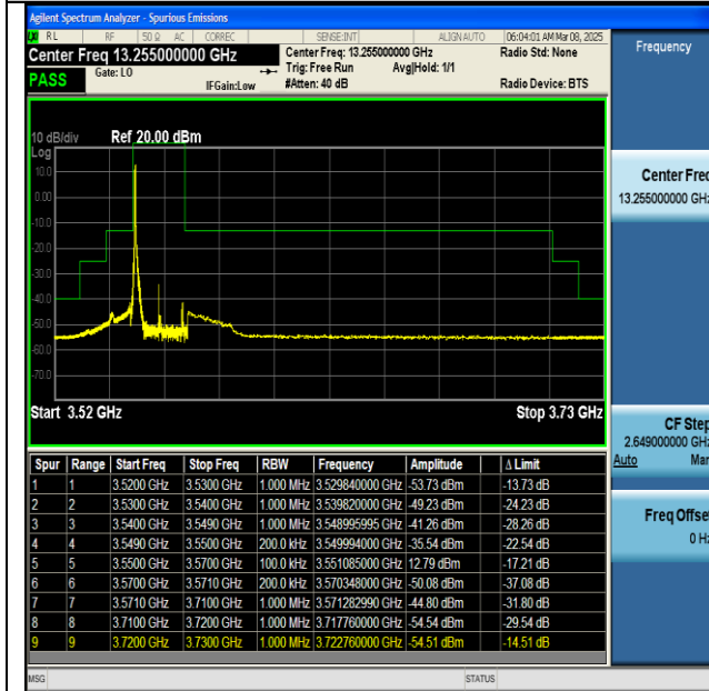
NTNV-n48-PC3-30-20-L-CP-QPSK-Edge_1RB_Left-PASS
