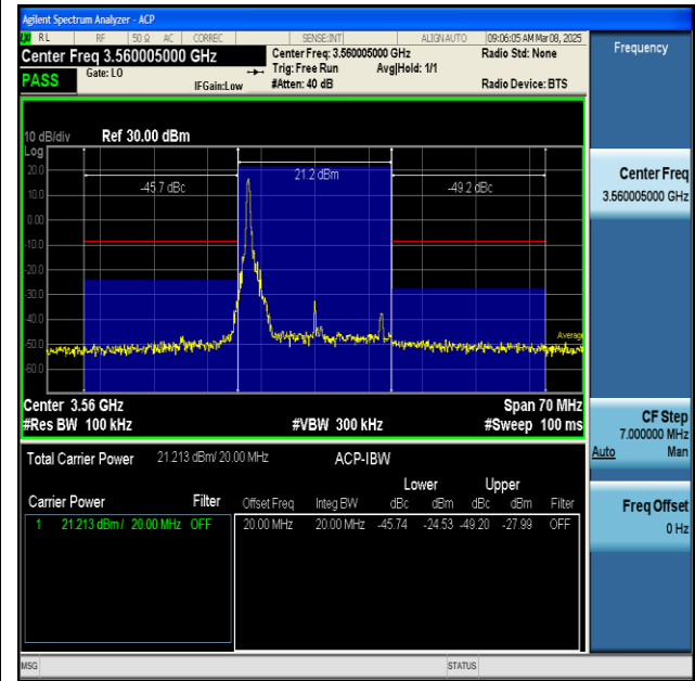
NTVN-n48-PC3-30-20-L-CP-QPSK-Inner_1RB_Left-PASS
