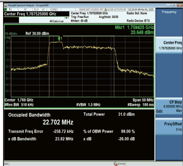
66-66-5MHz-20MHz-QPSK-QPSK-132455-132572- 25RB#0-100RB#0-PASS
