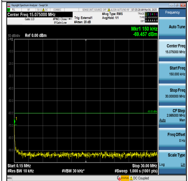
48-48-20MHz-20MHz-QPSK-QPSK-55891-56089-1RB#0- ORB#0-0.15~30MHz-PASS
