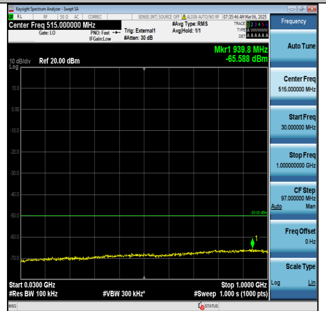
48-48-20MHz-20MHz-QPSK-QPSK-55891-56089-1RB#0- ORB#0-30~1000MHz-PASS
