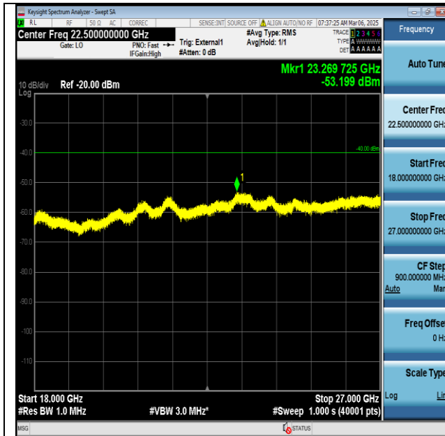
48-48-20MHz-20MHz-QPSK-QPSK-55891-56089-1RB#0- ORB#0-18000~27000MHz-PASS
