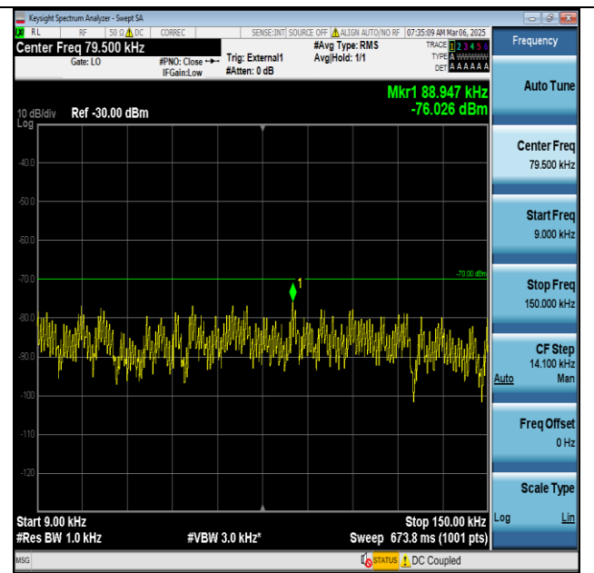
48-48-20MHz-20MHz-QPSK-QPSK-55891-56089-1RB#0- ORB#0-0.009~0.15MHz-PASS
