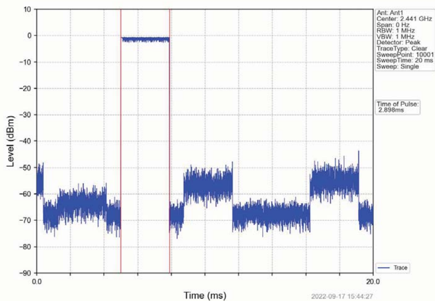
8DPSK_3DH5_HOPP_Ant1_NTNV
