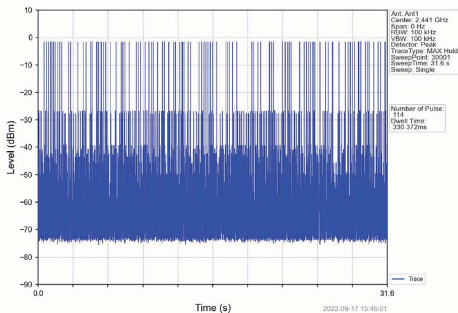
8DPSK_3DH5_HOPP_Ant1_NTNV
