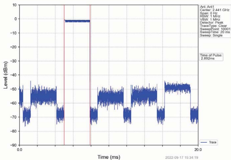
Pi/4DQPSK_2DH5_HOPP_Ant1_NTNV
