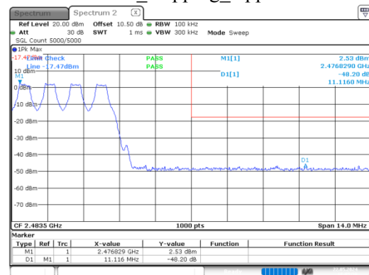
DH1_Hopping_Upper
