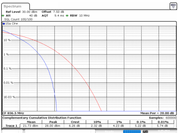
10MHz_Middle_QPSK_50@0
