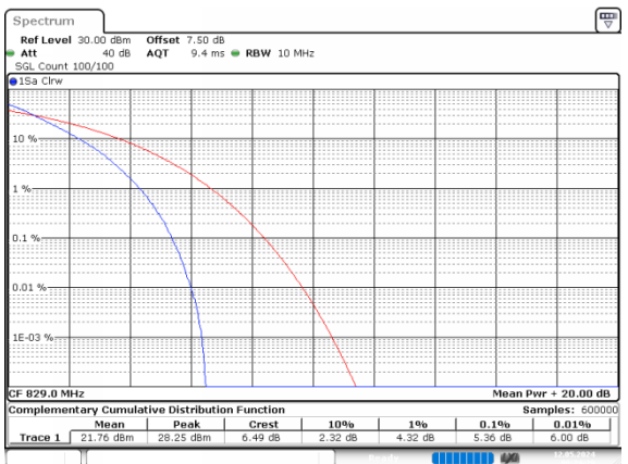
10MHz_Low_QPSK_50@0
