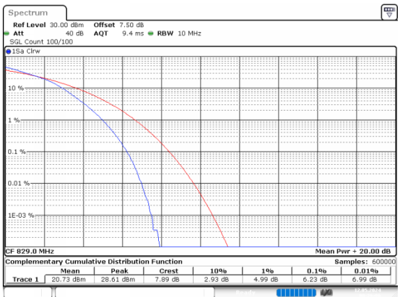
10MHz_Low_16QAM_50@0
