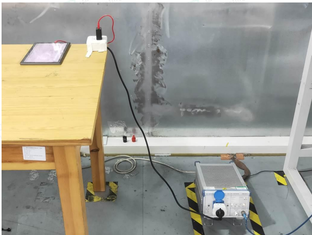
Fig. 3 DFS
