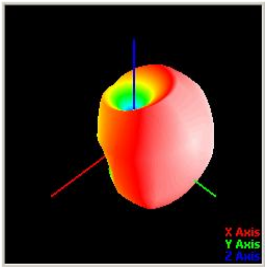
天线方向图
