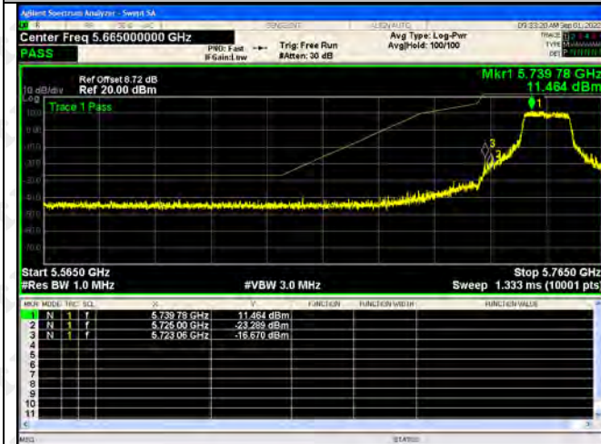
802.11(n20)-5745
