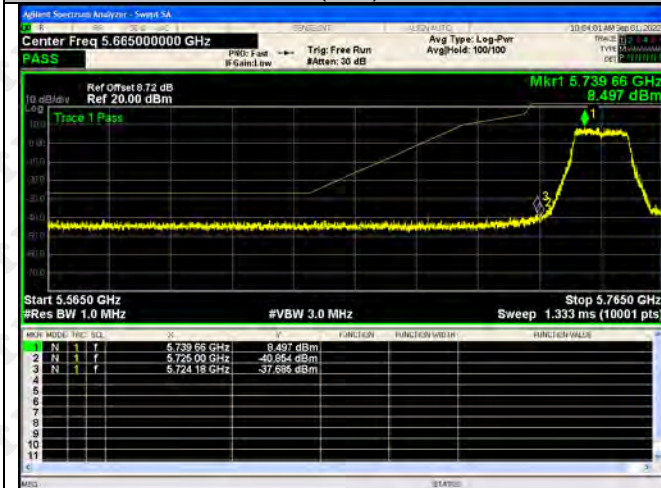
802.11(n40)-5755
