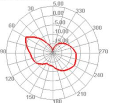
5100.000MHz H
