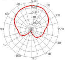
5100.000MHz E2
