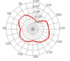
6000.000MHz H
