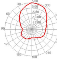
5550.000MHz E1
