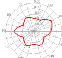
2500.000MHz E1
