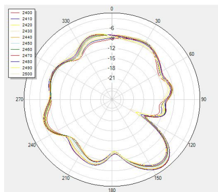
Phi=90
