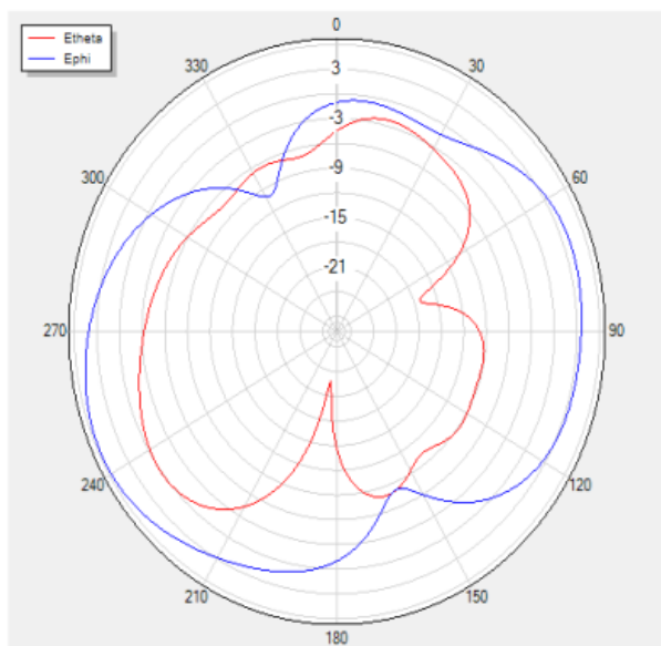
H Theta=90 freq=2400MHz
